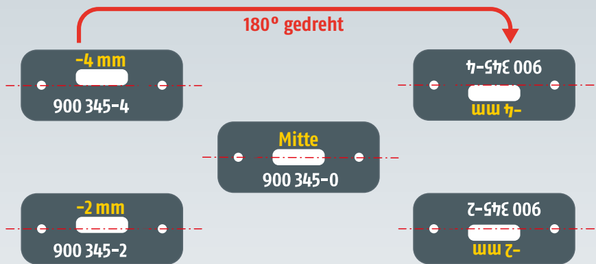
Verstellprinzip: 2 Basisschrauben mit 3 Bodenmulden = 5 verschiedene Lochpositionen
