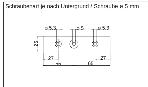
Art. No. 1-405 Zapfenband-Oberteil DIN Links und Rechts verwendbar, mit Polyamidbuchse, horizontal justierbar Art. No. 1-405 Top off-set usable for left or right handed doors, with polyamide sleeve, adjustable in horizontal direction
