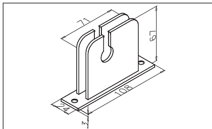
Art. No. 2-623 Riegelschloss für Türschiene oben oder unten Art. No. 2-623 bolt lock for upper or lower door rail
