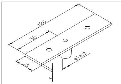
Art. No. 1-110 PT 24 Anschraubplatte mit Bolzen, ohne Schrauben Max. Flügelgewicht: 80 kg Art. No. 1-110 PT 24 Fixing plate with pivot, without screws max. weight per wing: 80 kg
