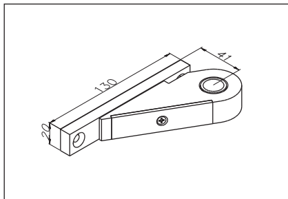
Art. No. 1-405 Zapfenband-Oberteil DIN Links und Rechts verwendbar, mit Polyamidbuchse, horizontal justierbar Art. No. 1-405 Top off-set usable for left or right handed doors, with polyamide sleeve, adjustable in horizontal direction
