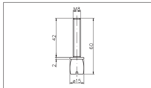
Art. No. 1-117 PT 25 Bolzen mit Messingdübel M8, passend zu oberer Türschiene
