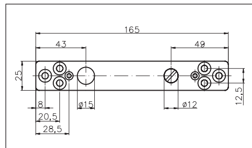
Art. No. 1-115 PT 21 Zapfen mit hochdrehbarem Bolzen, ohne Schrauben
