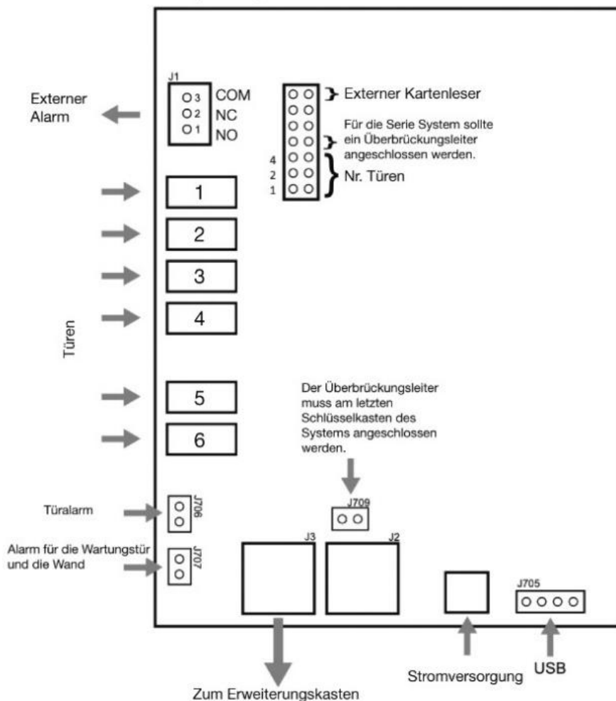
Leiterplatte - System
