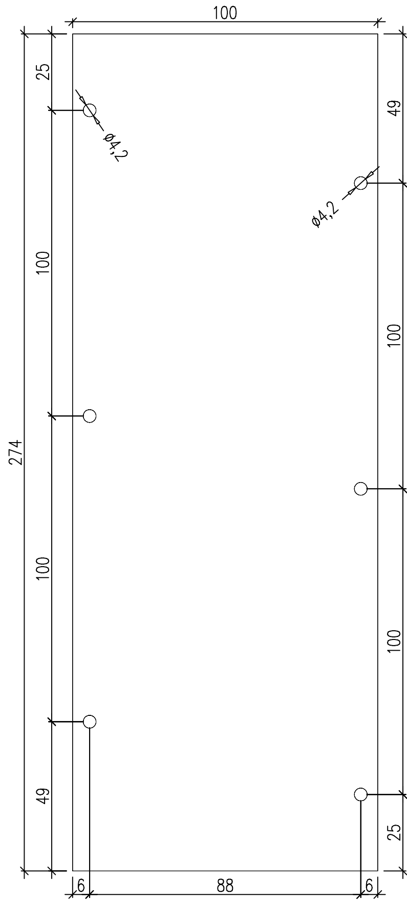
Draufsicht
