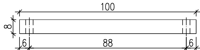
Draufsicht
