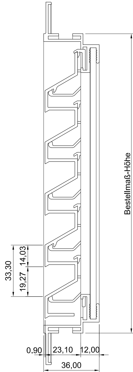
Draufsicht
