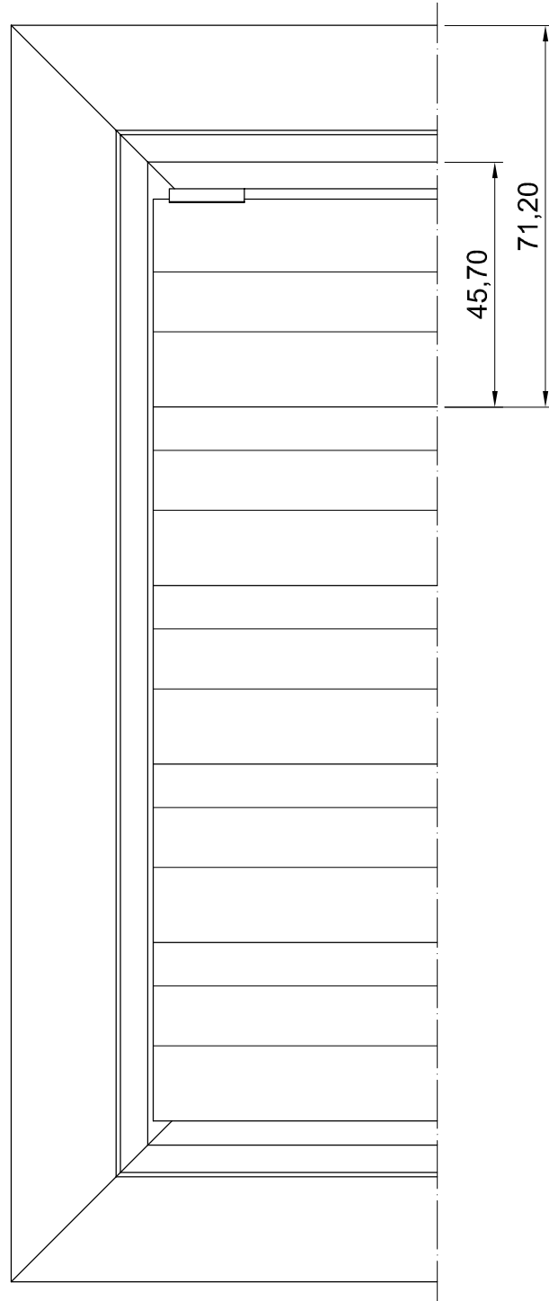
Seitenansicht
