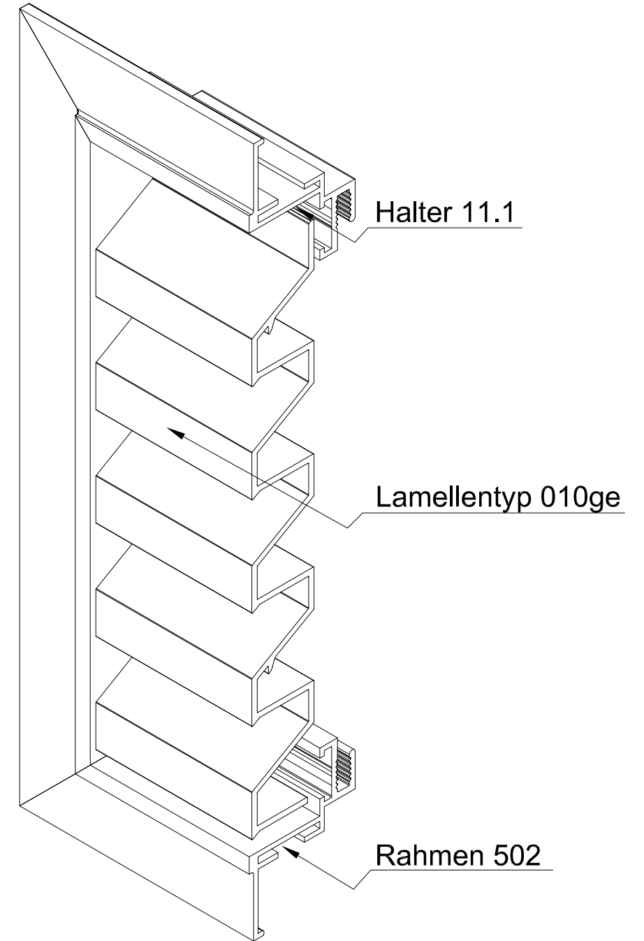
ISO-Ansicht
