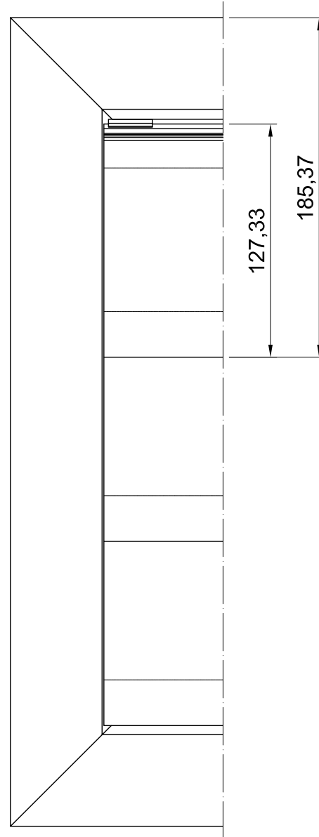
Vorderansicht
