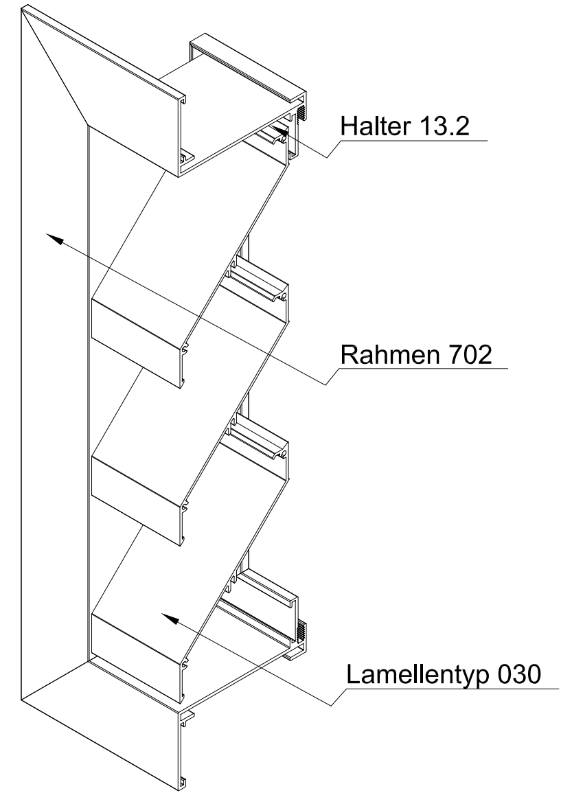
ISO-Ansicht
