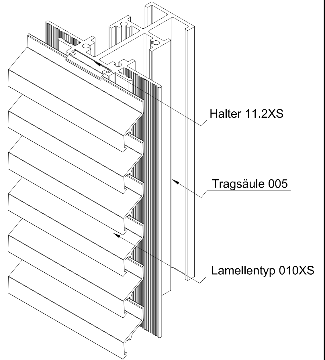
ISO-Ansicht
