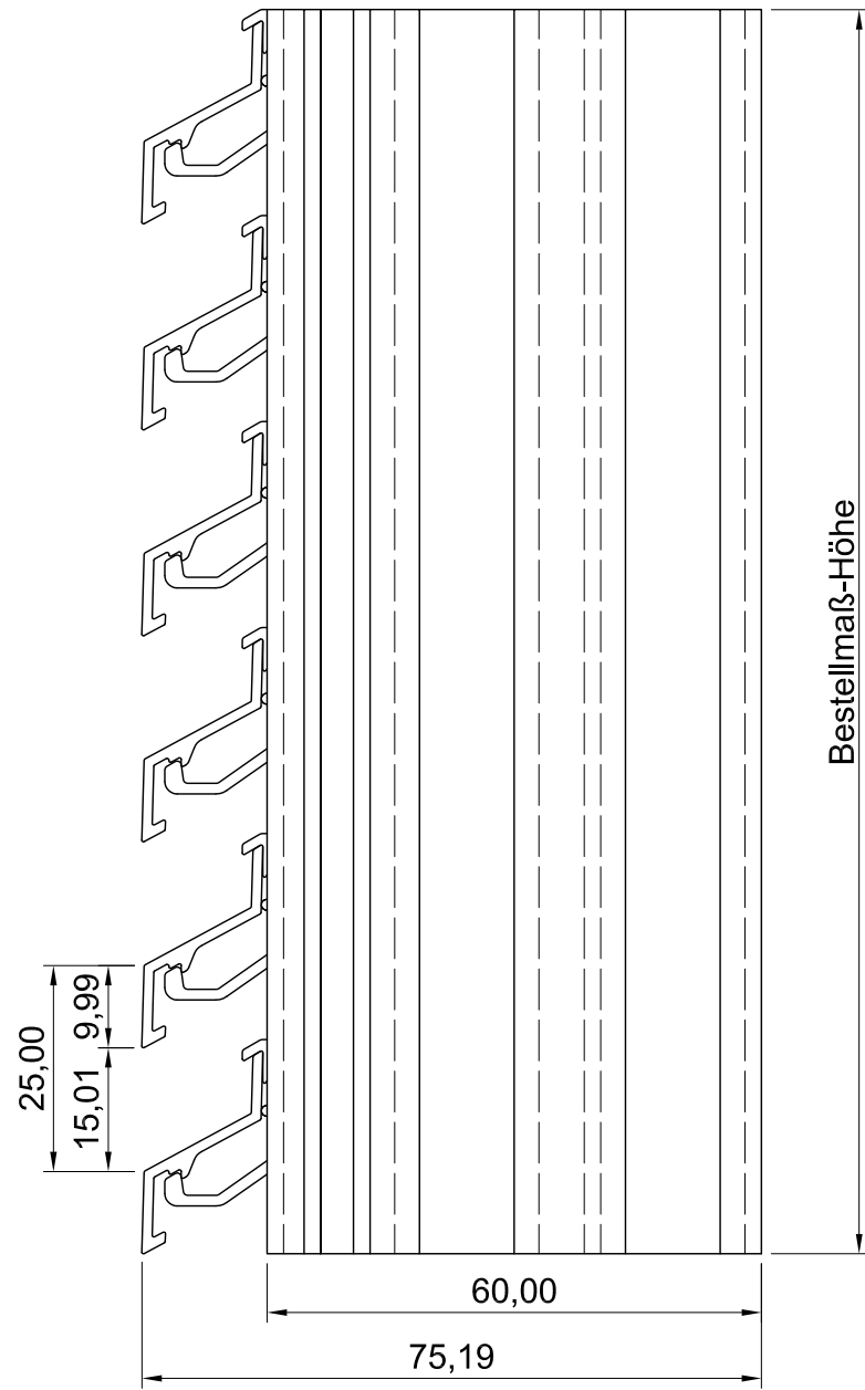
Draufsicht
