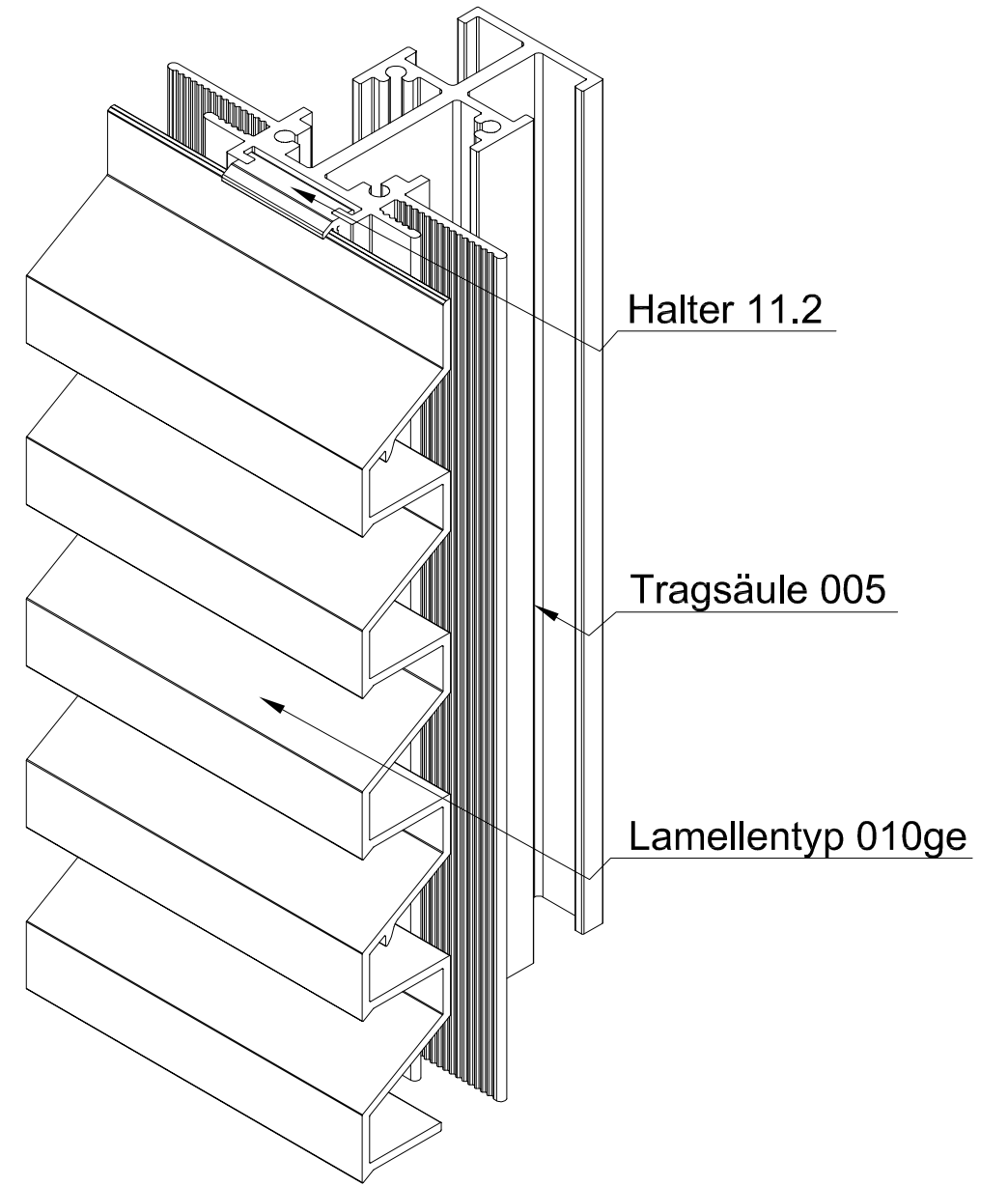
ISO-Ansicht
