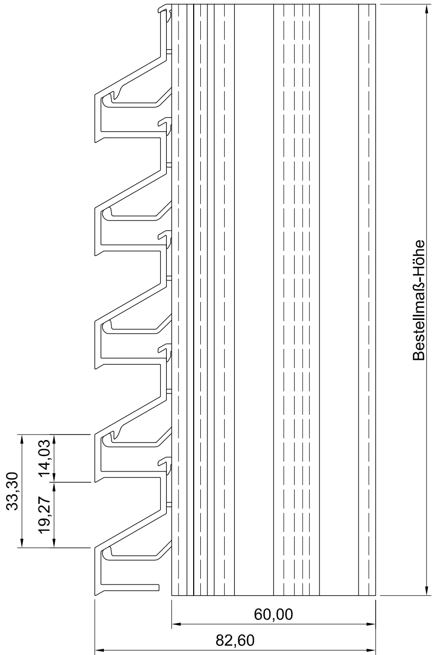
Draufsicht
