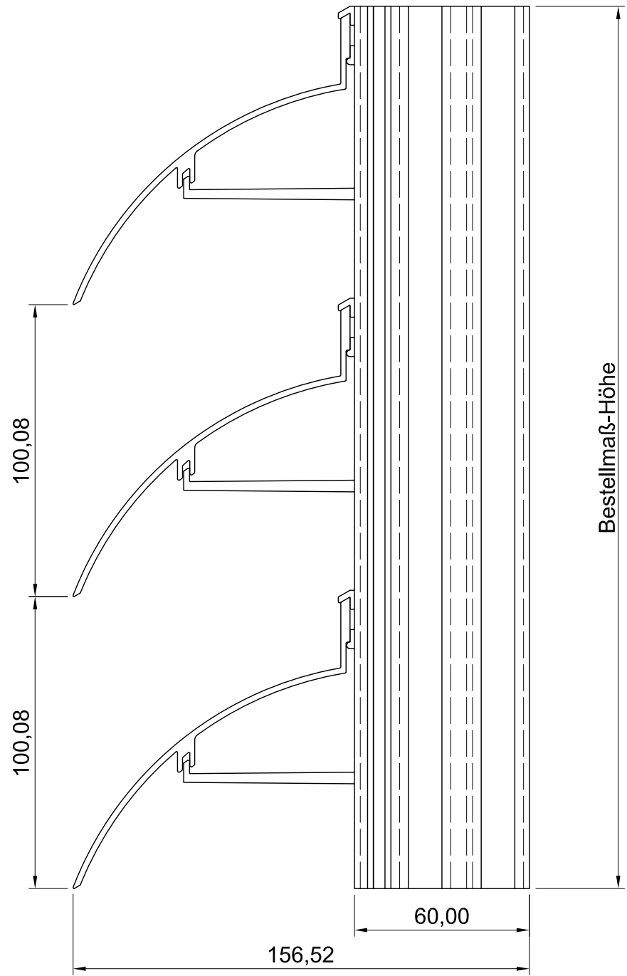
Seitenansicht
