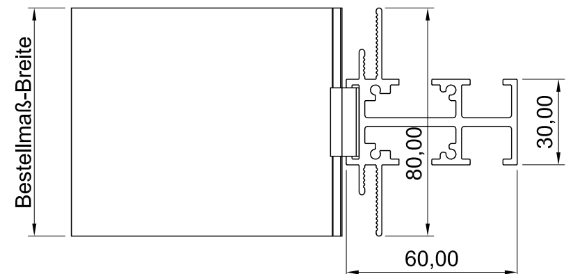
Draufsicht
