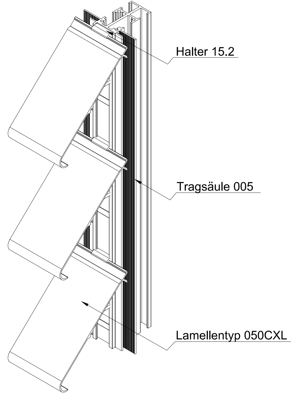
ISO-Ansicht
