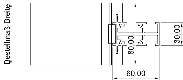
Draufsicht
