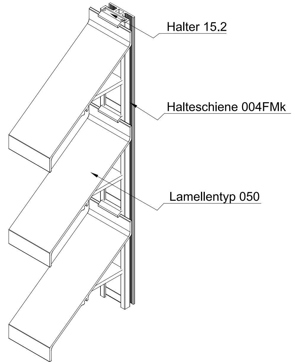
ISO-Ansicht
