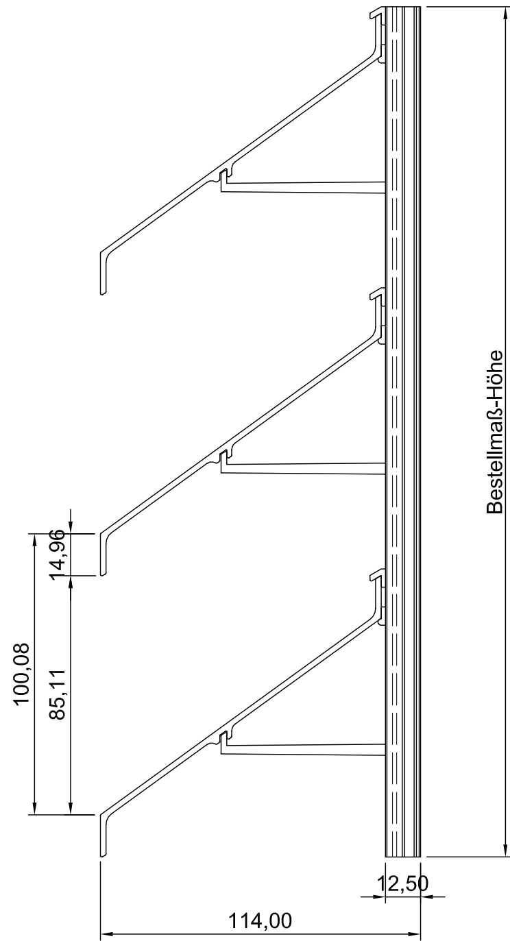
Seitenansicht
