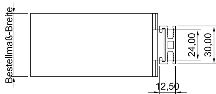
Draufsicht
