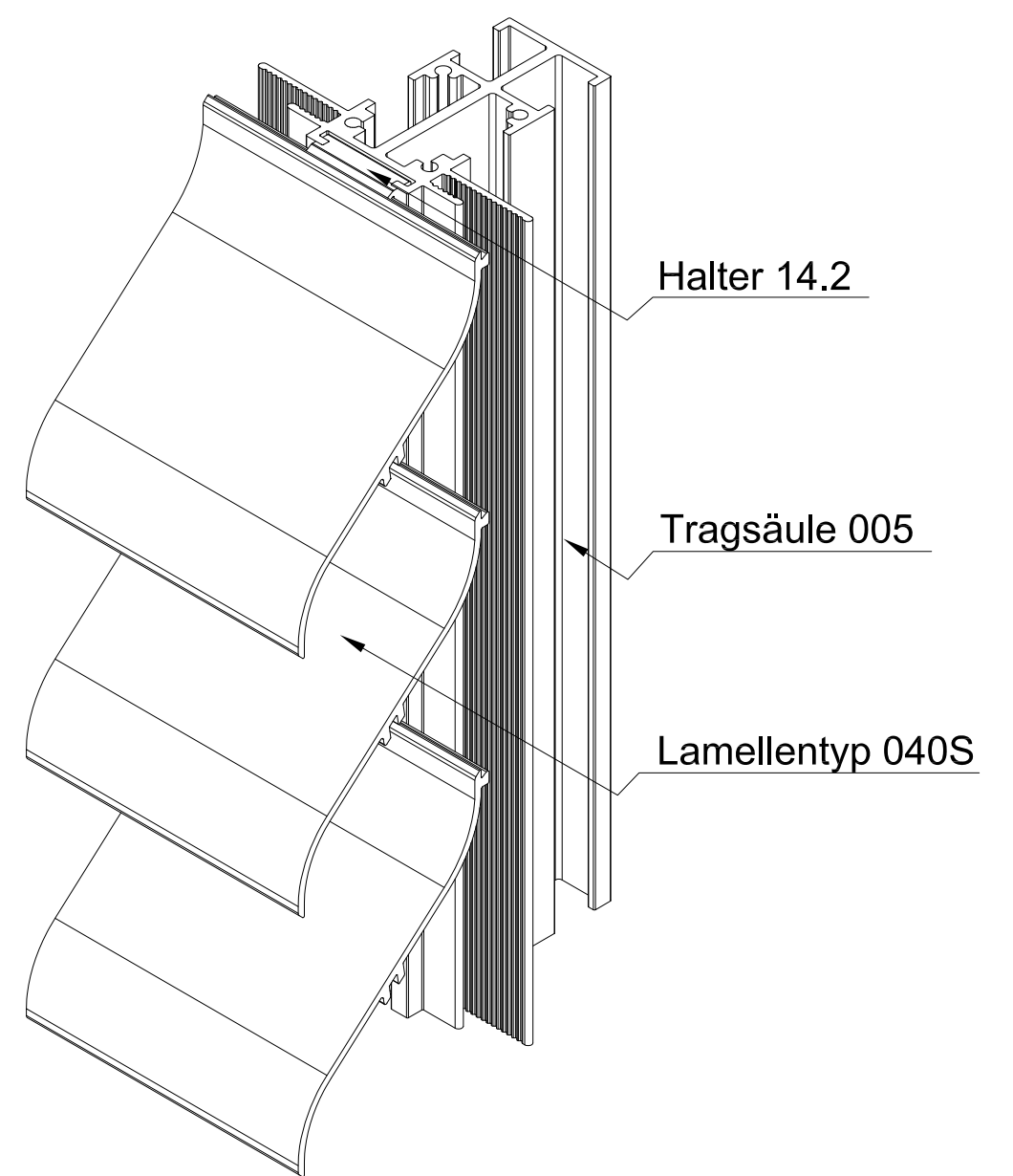
ISO-Ansicht
