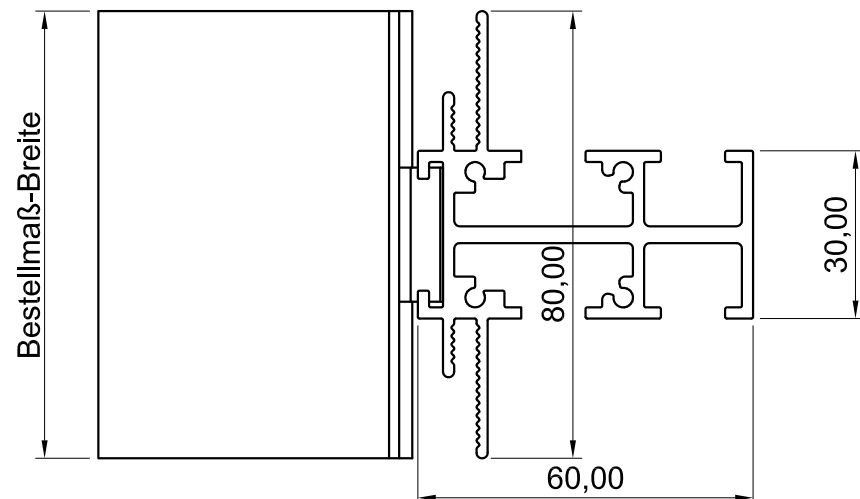
Draufsicht
