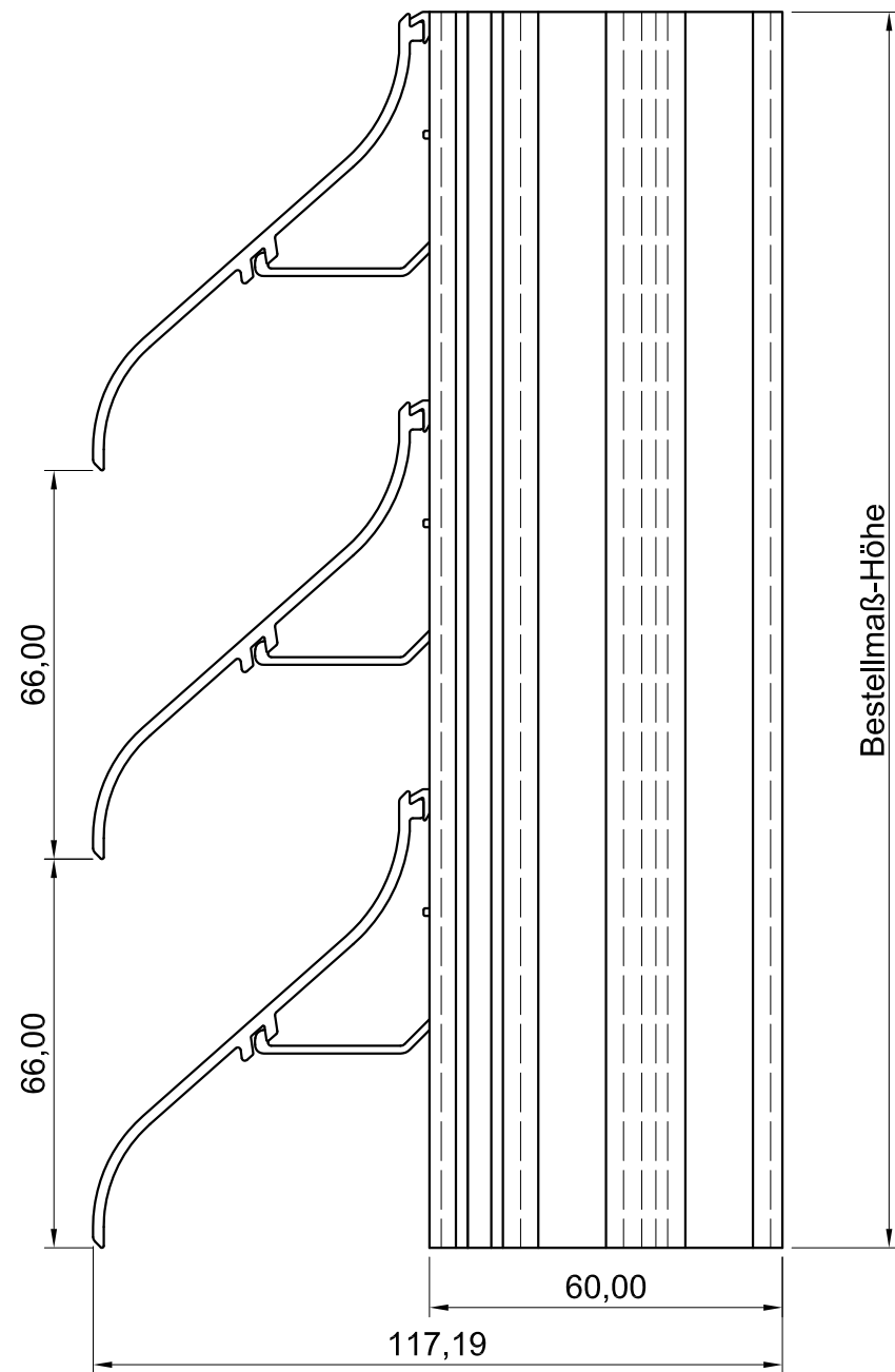
Draufsicht
