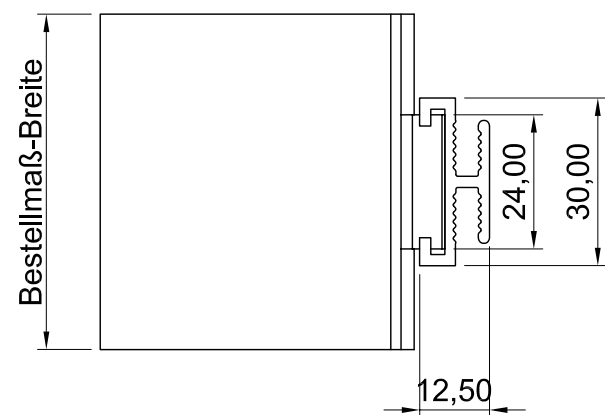
Draufsicht
