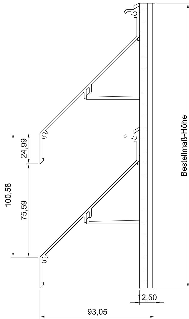
Seitenansicht
