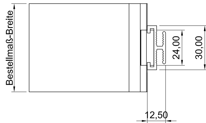
Draufsicht
