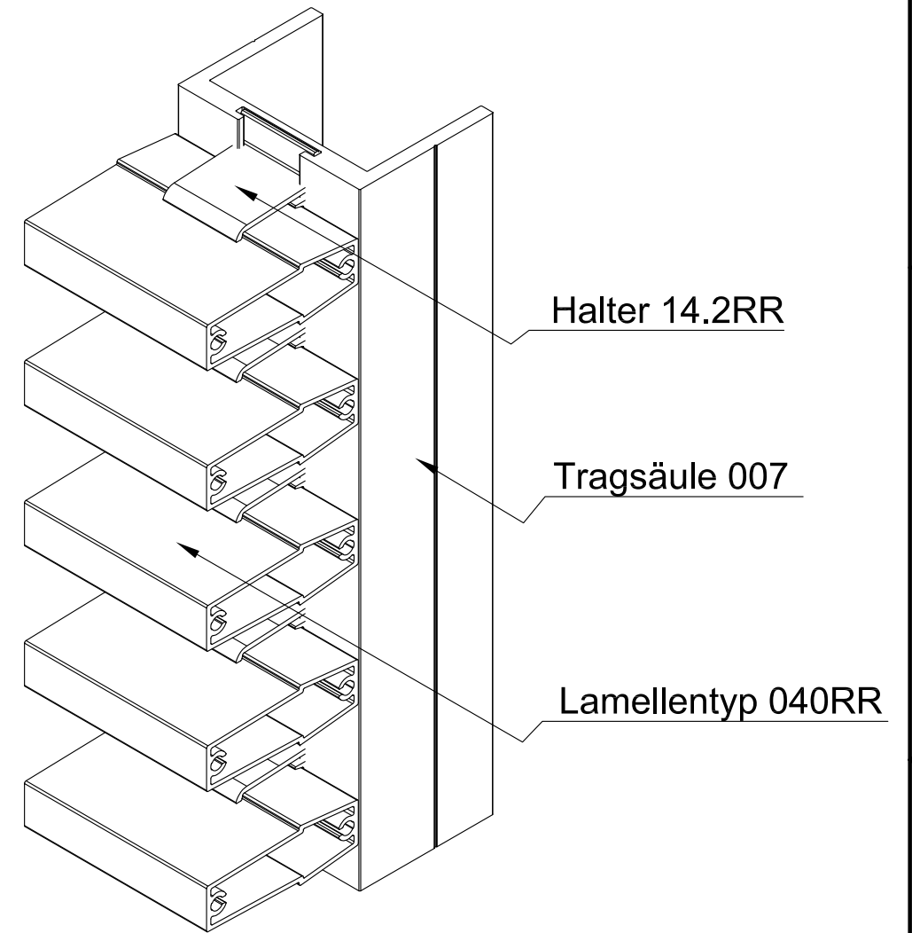
ISO-Ansicht
