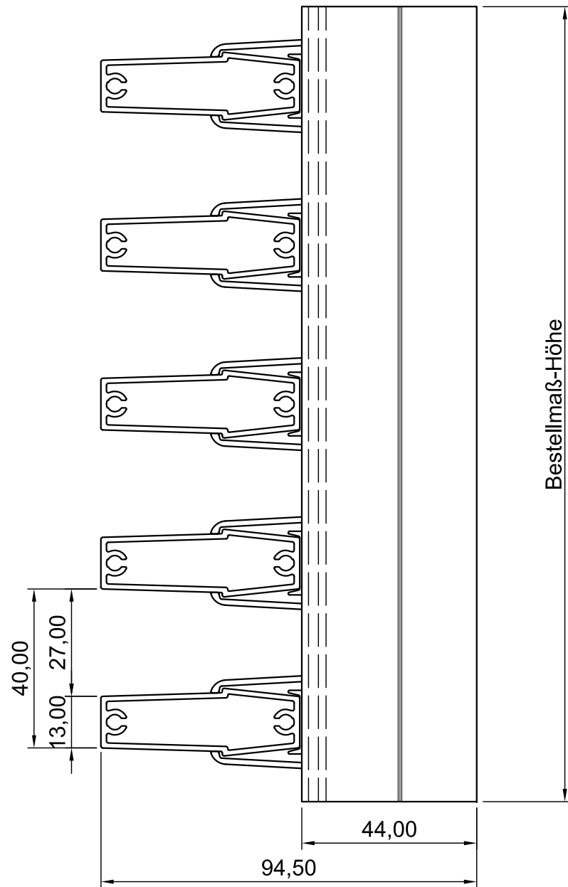
Seitenansicht
