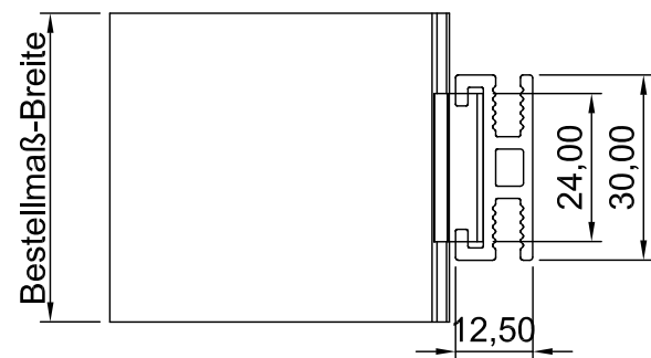
Draufsicht
