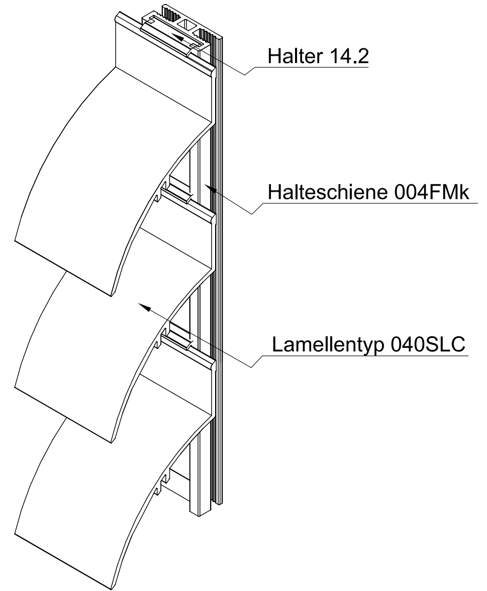
ISO-Ansicht
