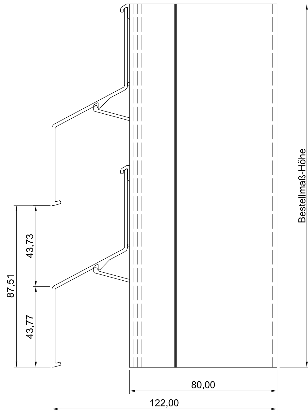
Draufsicht
