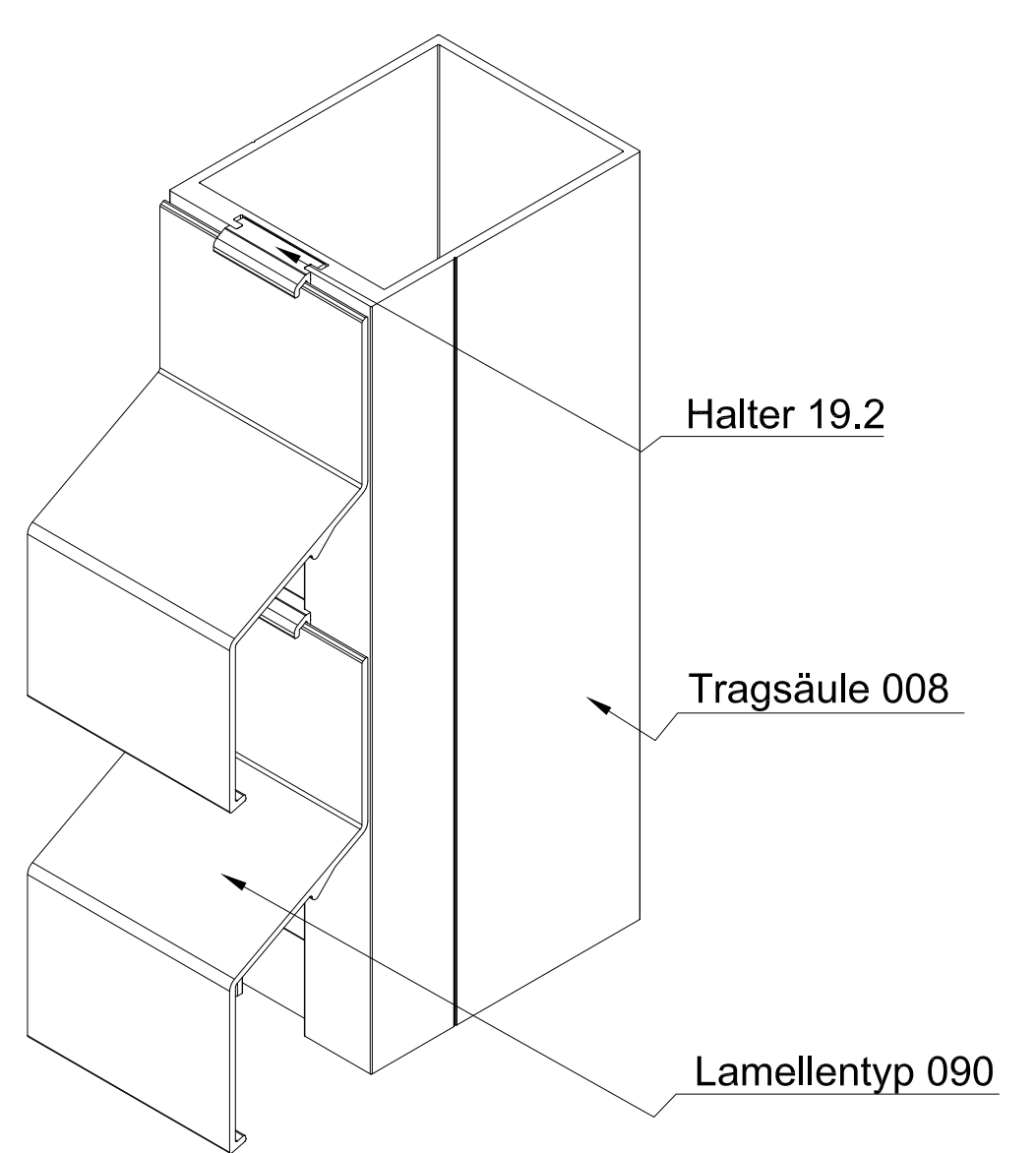
ISO-Ansicht
