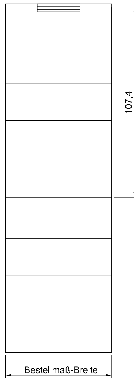
Vorderansicht
