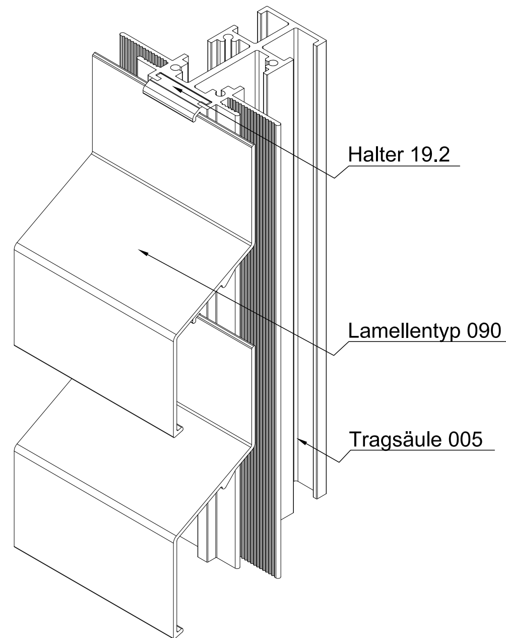
ISO-Ansicht
