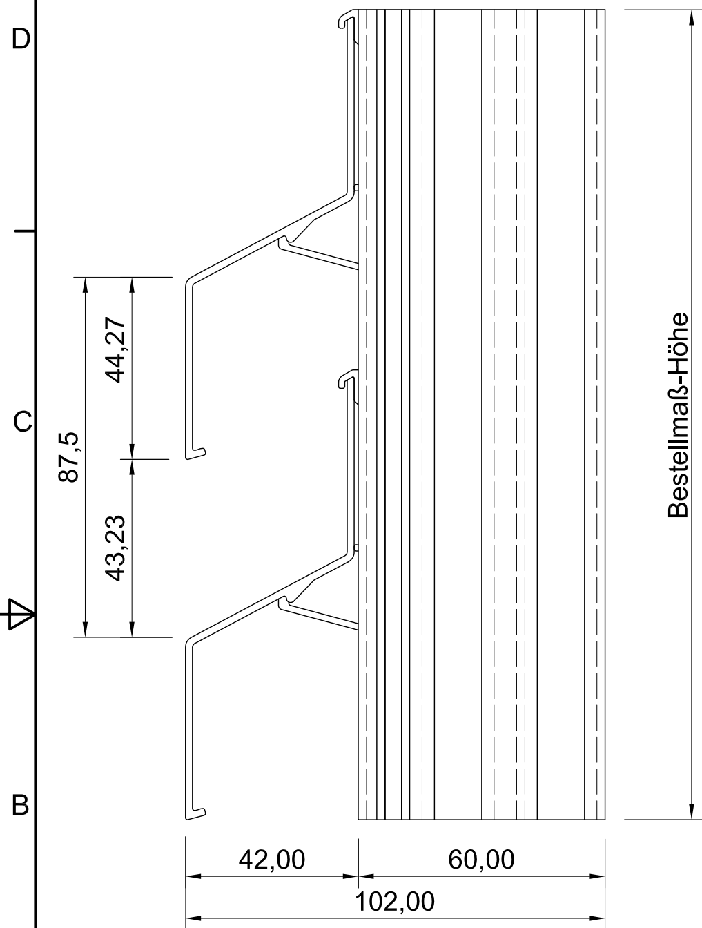
Seitenansicht
