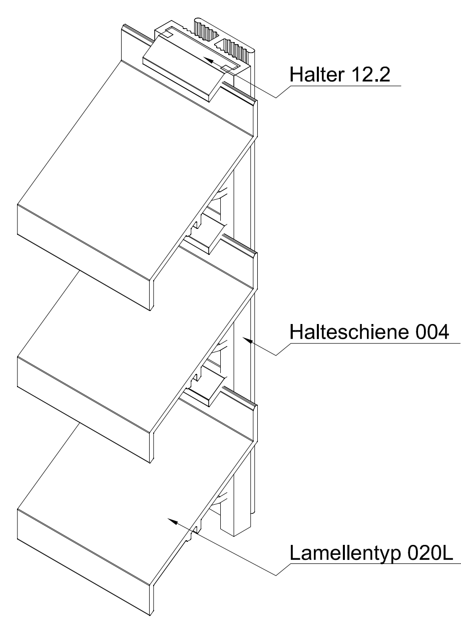
ISO-Ansicht
