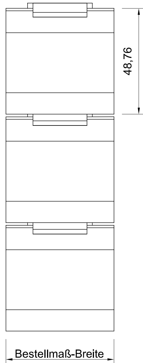
Seitenansicht
