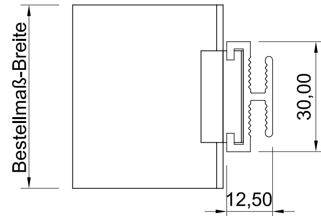
Draufsicht
