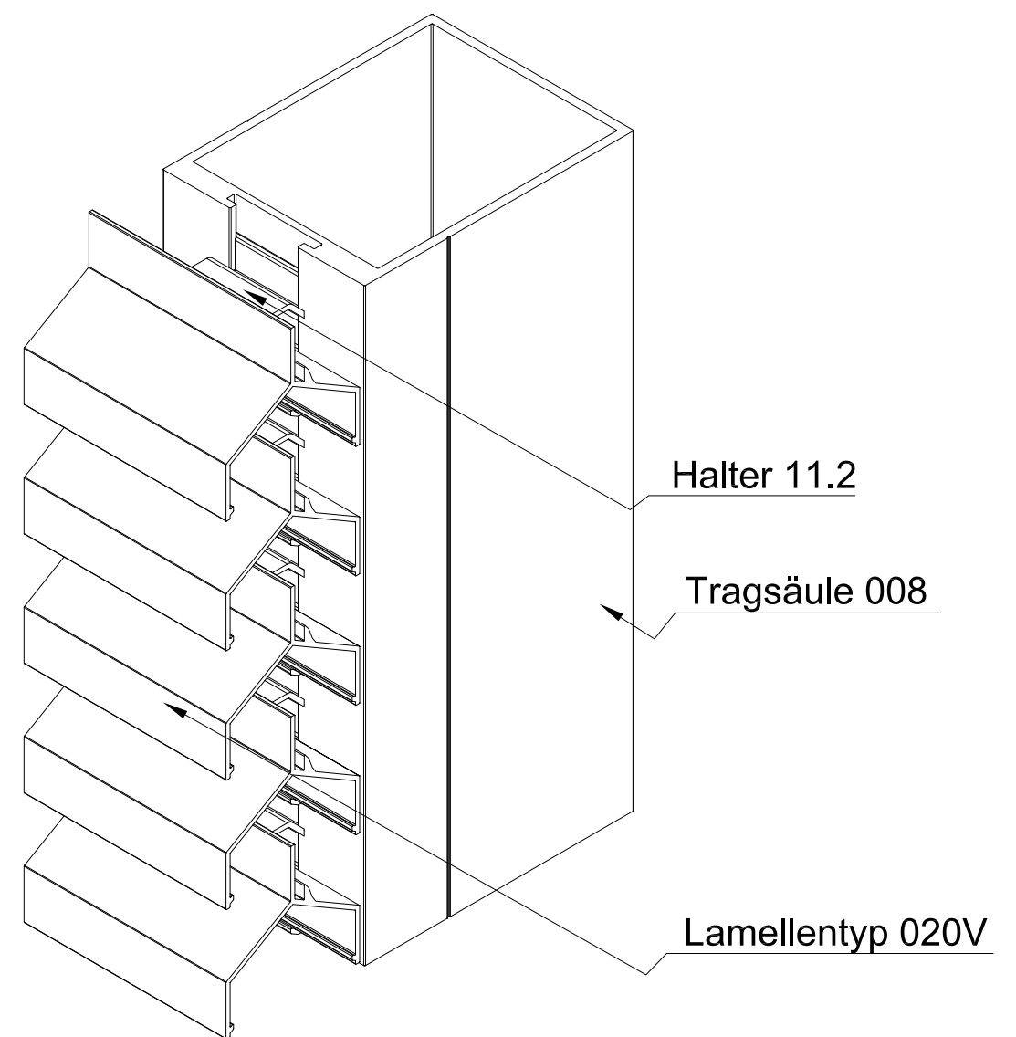
ISO-Ansicht
