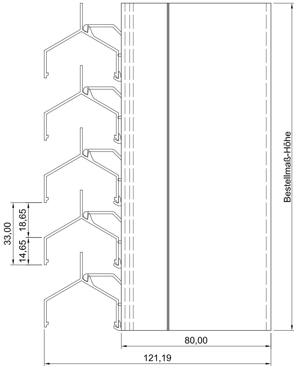
Draufsicht
