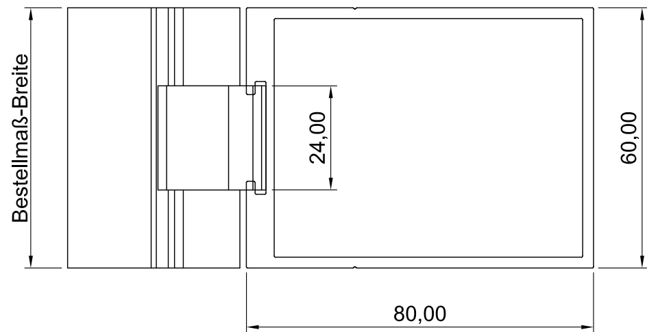
Draufsicht
