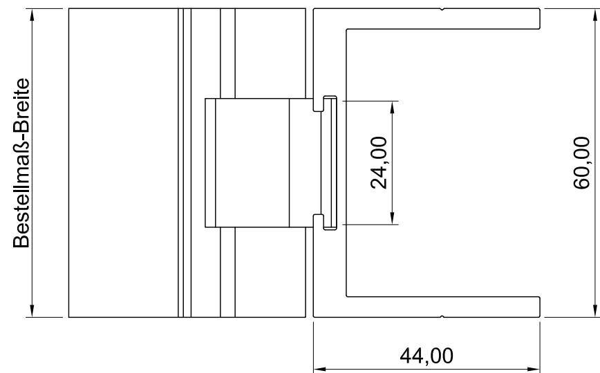
Draufsicht
