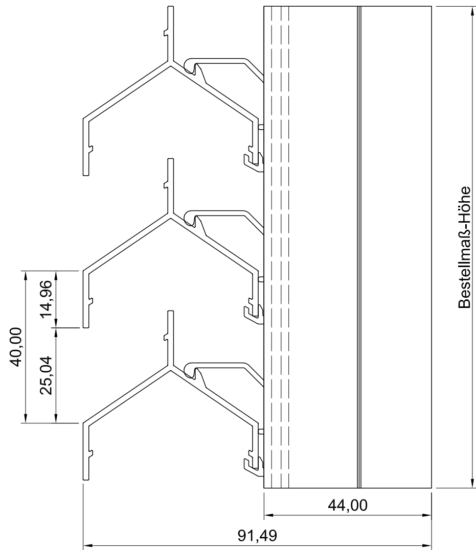
Seitenansicht
