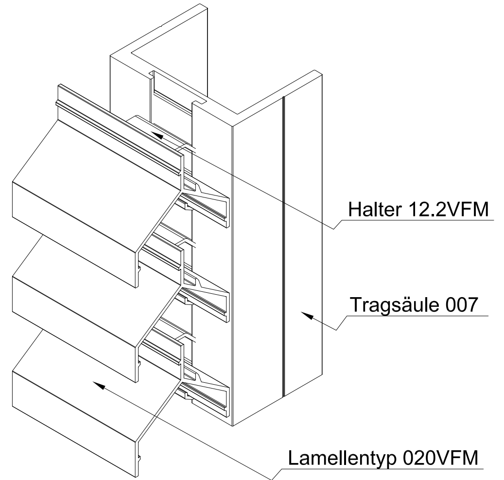
ISO-Ansicht
