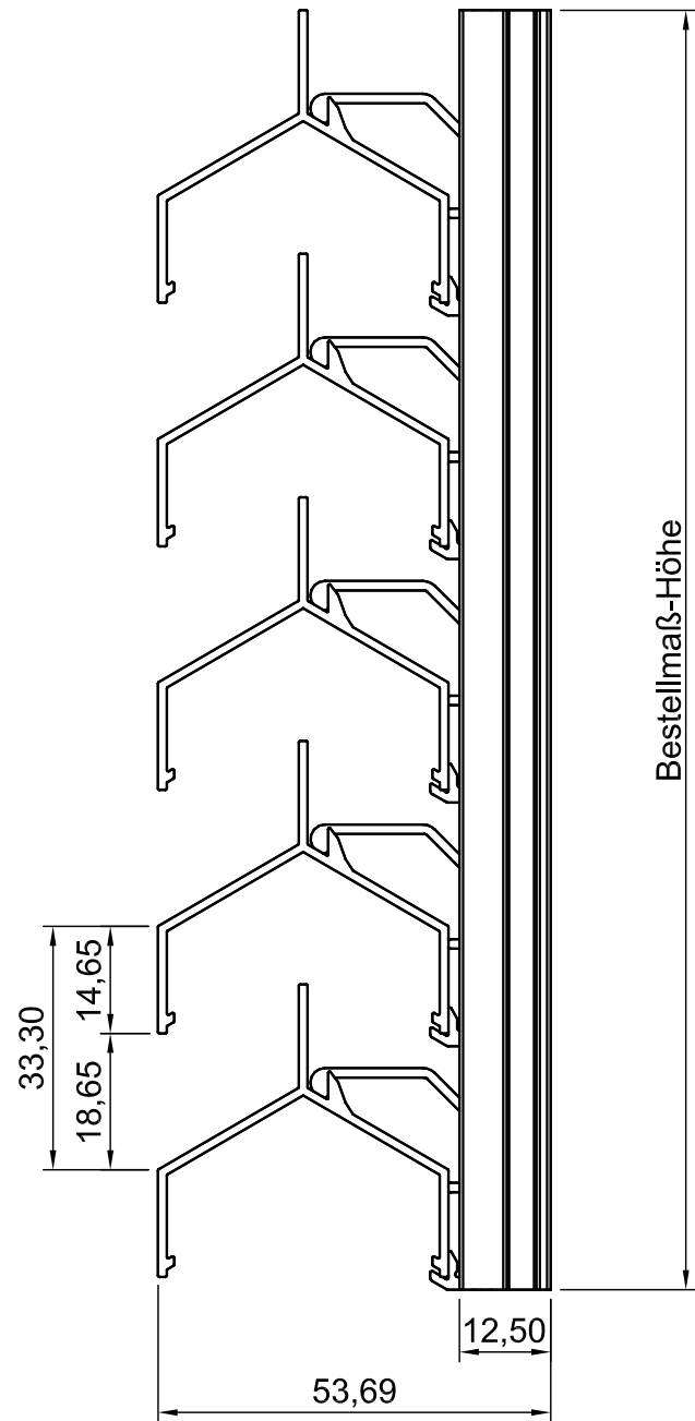
Draufsicht
