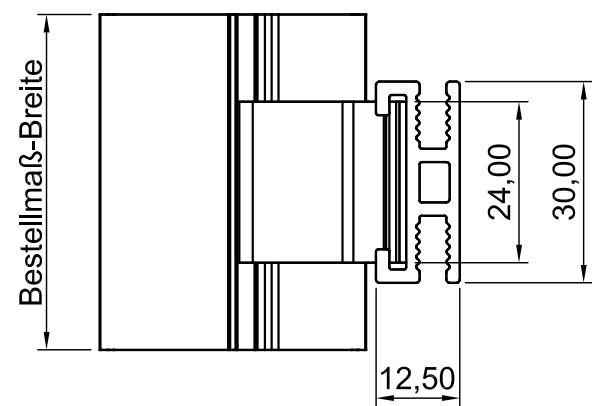
Draufsicht
