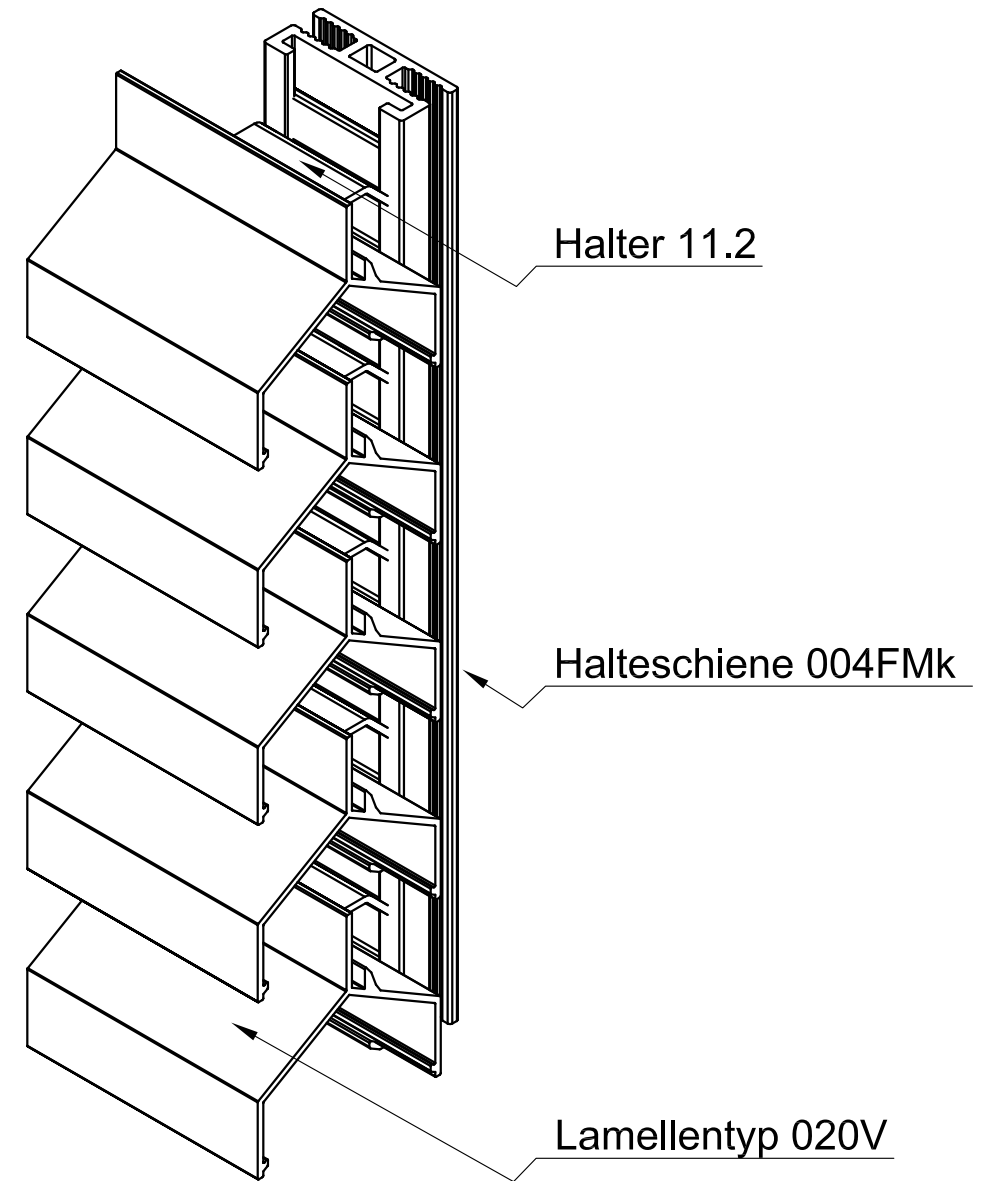
ISO-Ansicht
