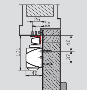
Sturzfutterwinkel Zum Anbringen der Gleit- schiene an Türrahmen mit tiefem Sturz bei Montage auf der Bandgegenseite.
