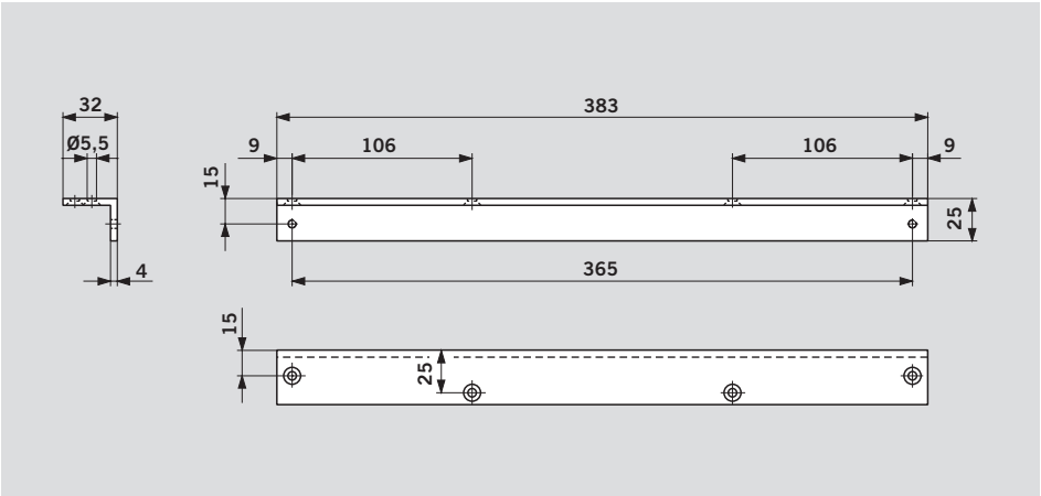
Sturzfutterwinkel Zum Anbringen der Gleit- schiene an Türrahmen mit tiefem Sturz bei Montage auf der Bandgegenseite.
