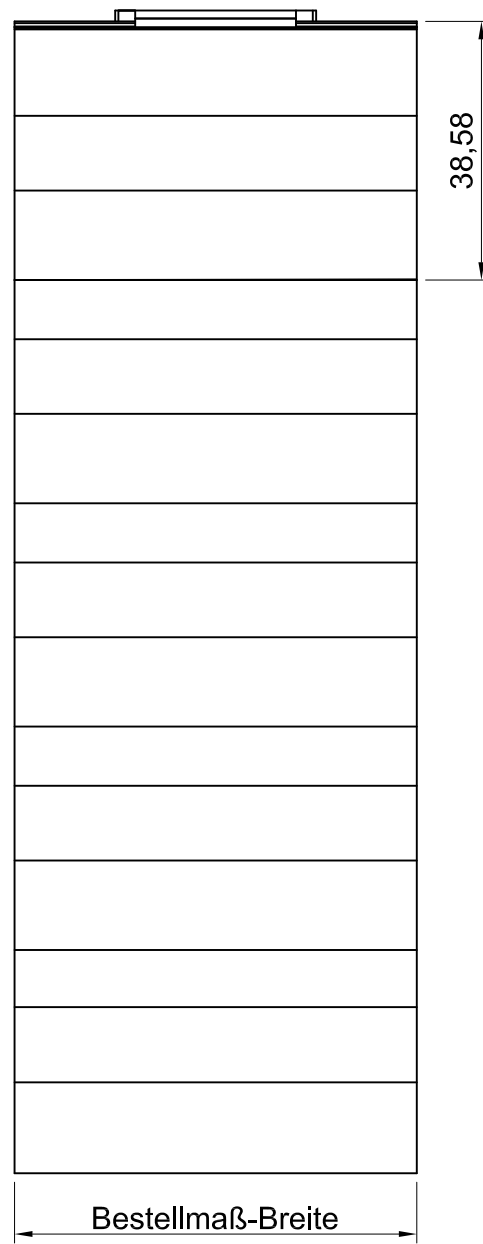
Vorderansicht
