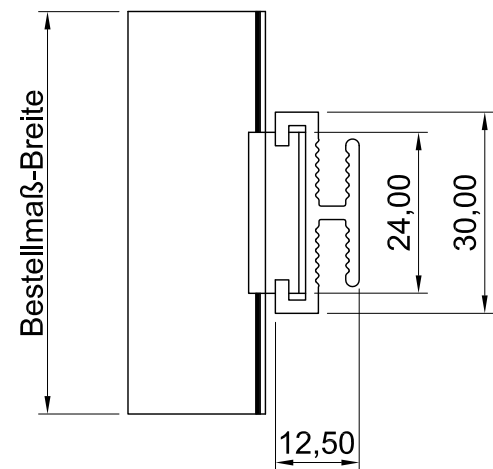
Draufsicht
