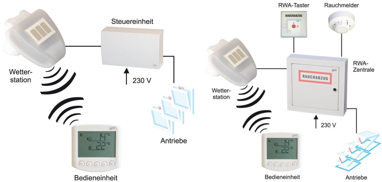
10.5.a Mit WUC- / WCC- Steuerung
