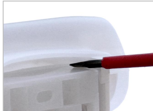
6.2.2.b Schieben Sie den Halter nach unten heraus eines Schraubendrehers
