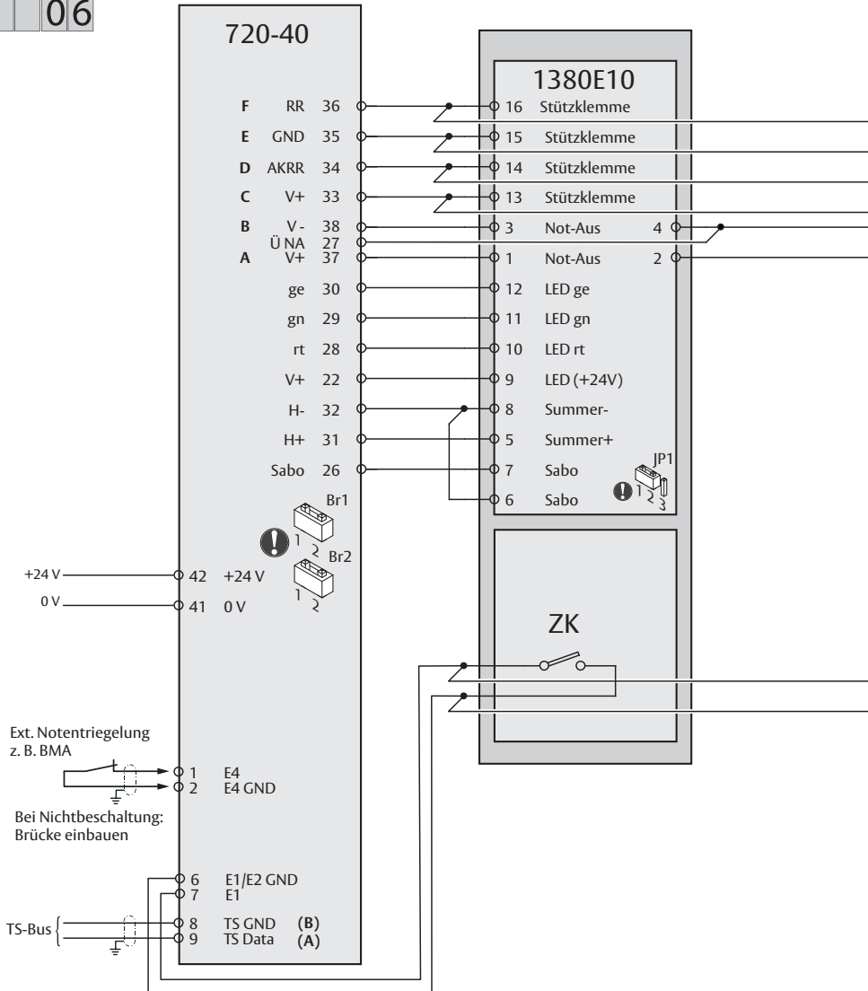
AP001300: 1380E10 mit Bedienung über Zutrittskontrolle
