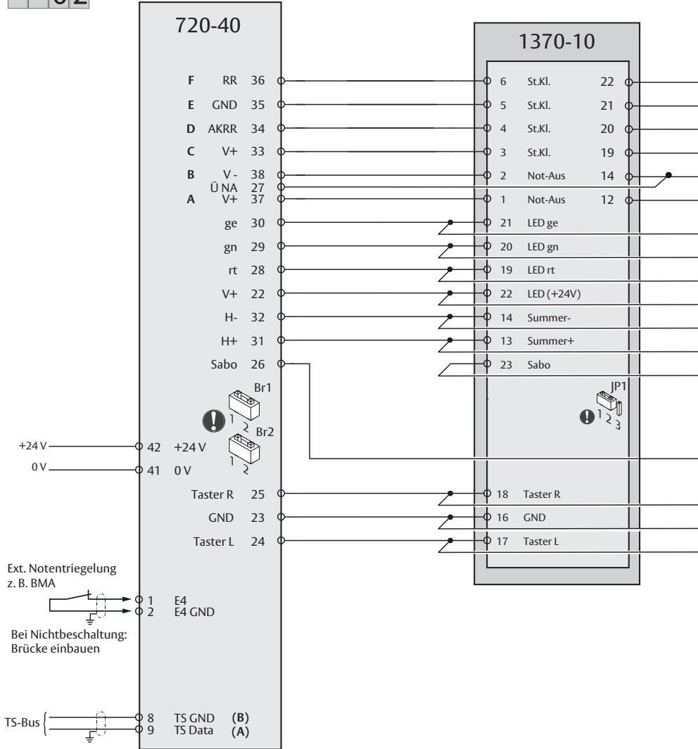
AP001000: 1370-10 mit Schlüsselschalter auf der Außenseite
