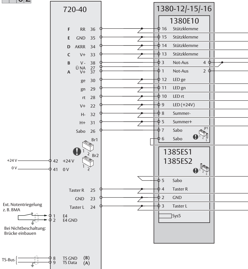
AP000601: 1380-12/-15/-16 mit Schlüsselschalter auf der Außenseite
