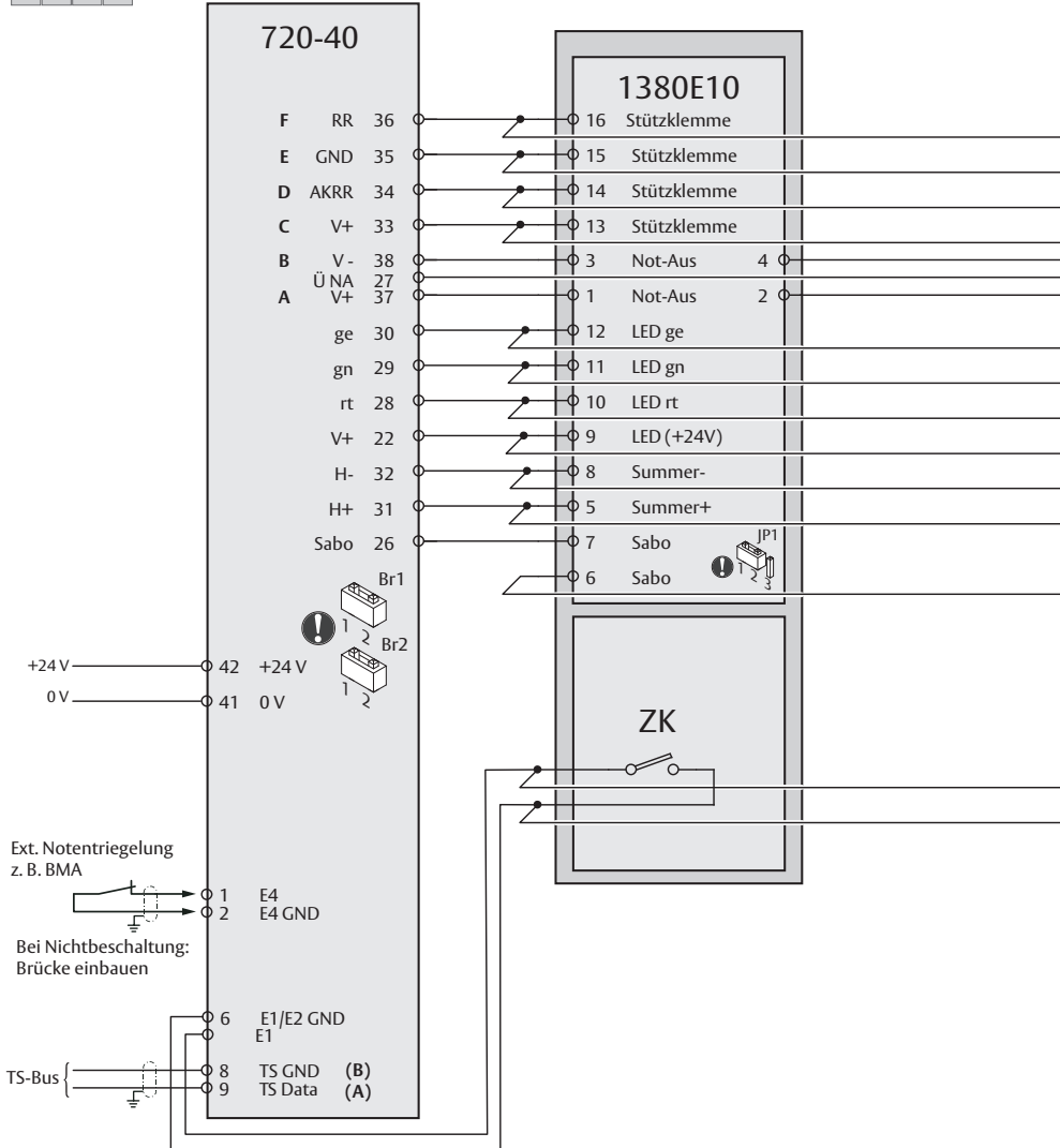
AP001900: 1380E10 beidseitig mit Bedienung über Zutrittskontrolle
