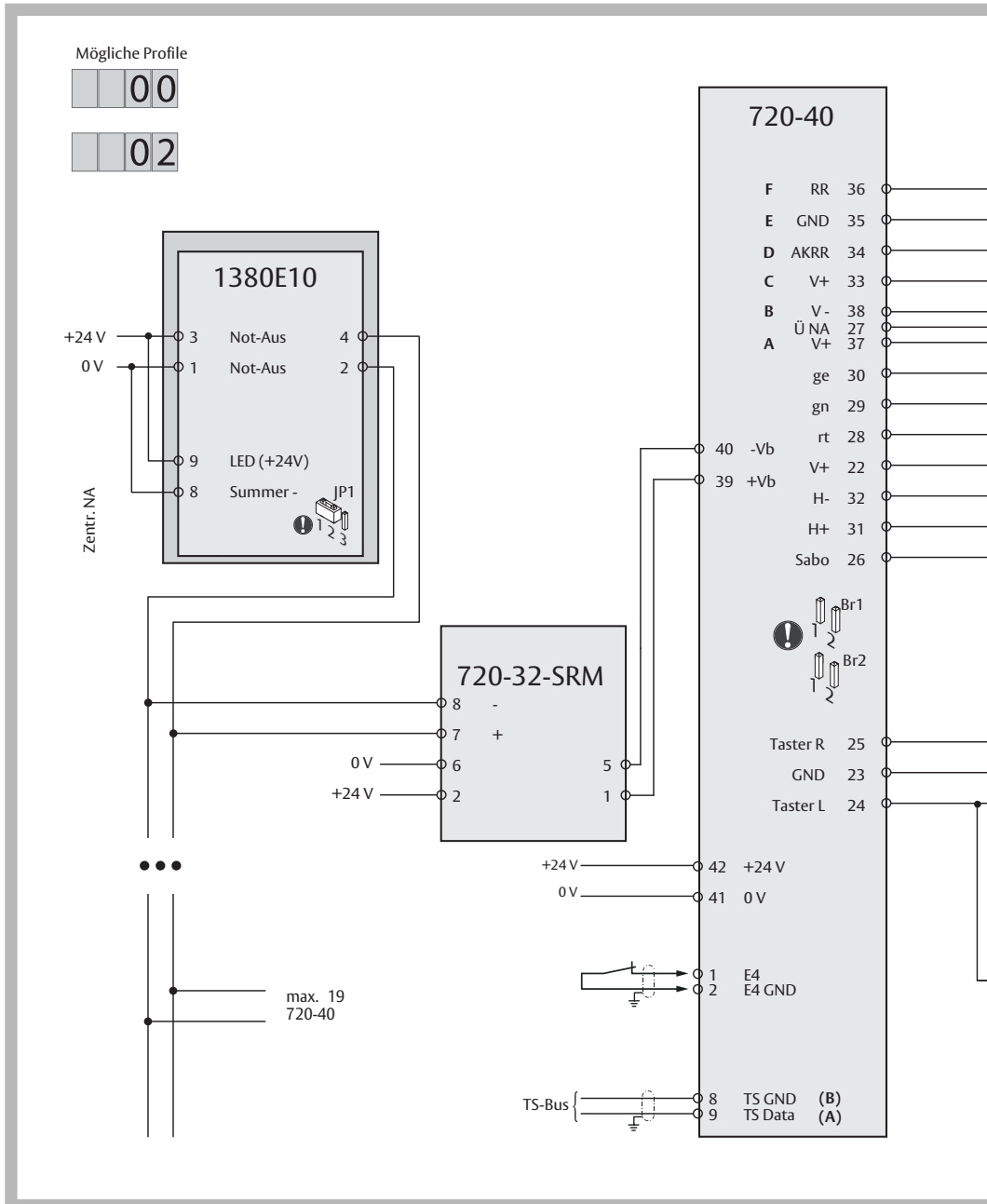
AP003400: 1380-12/-16 mit Schlüsselschalter entgegen der Fluchrichtung (Innenbereich)
