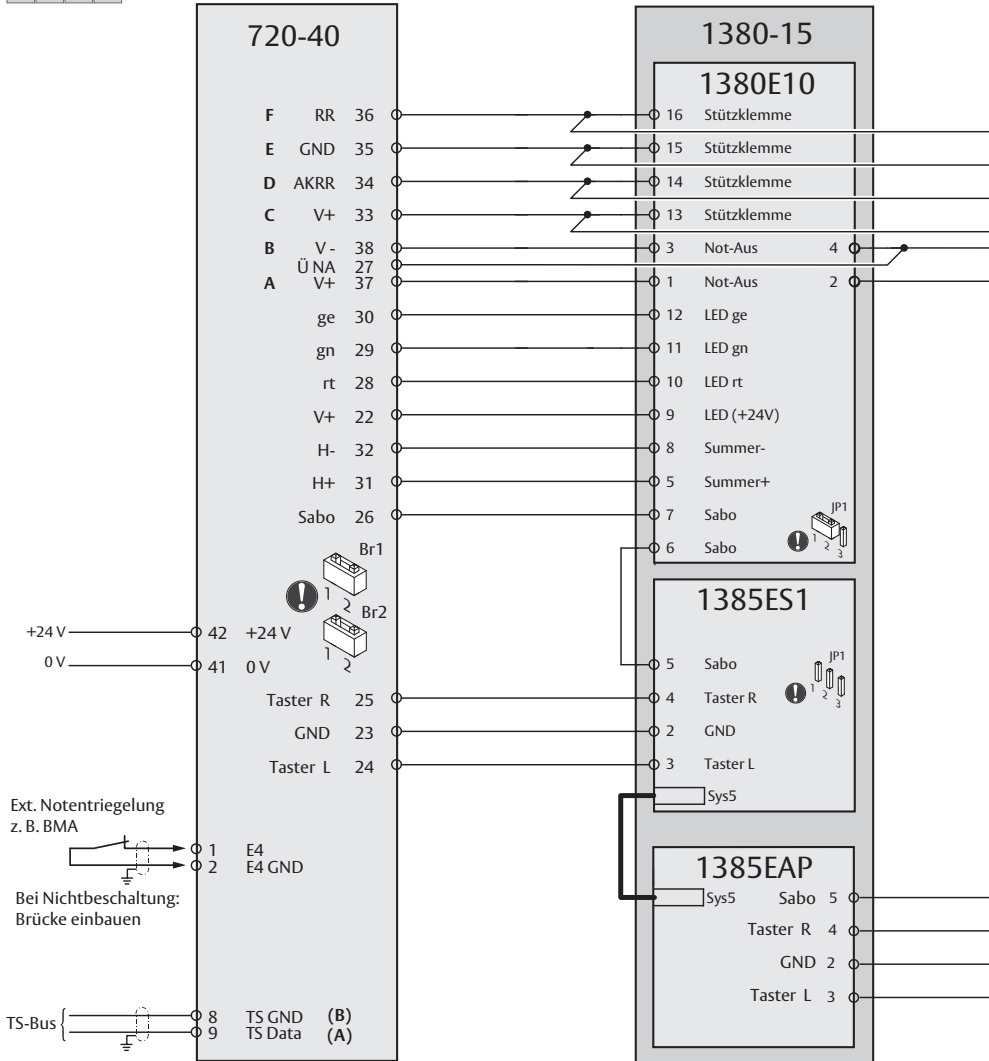
AP000501: 1380-15 mit Schlüsselschalter entgegen der Fluchrichtung (Innenbereich)
