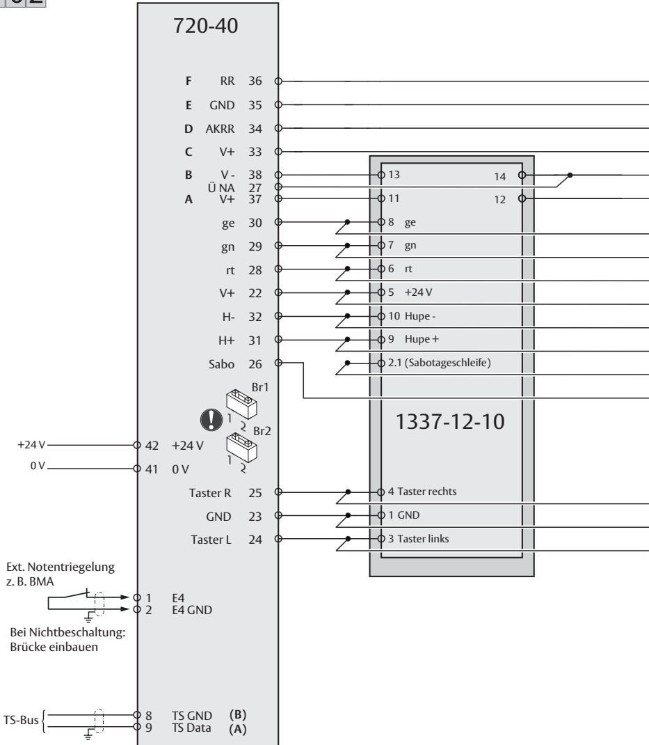
AP001200: 1337-12 mit Schlüsselschalter entgegen der Fluchtrichtung
