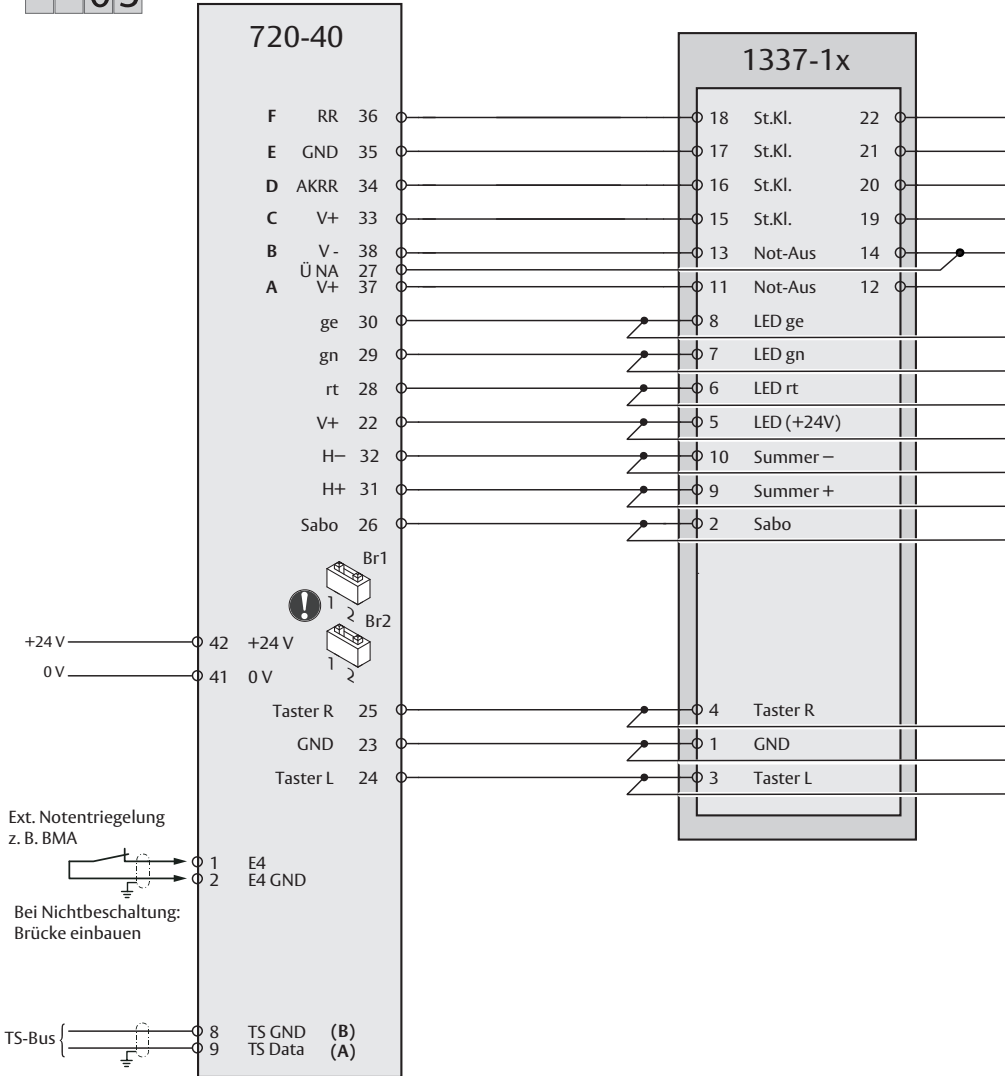
AP000800: 1337-10/-11 mit Schlüsselschalter auf der Außenseite
