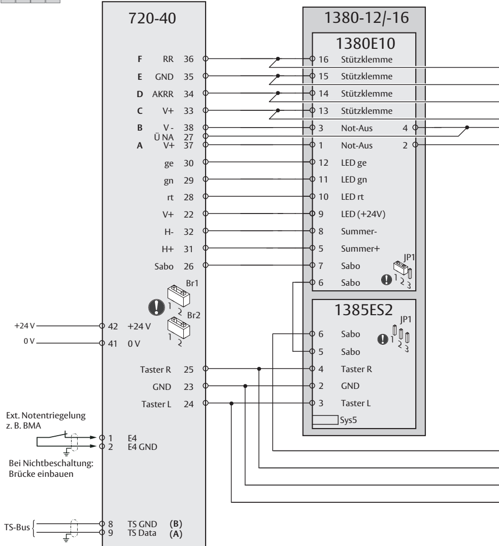
AP003100: 1380-12/-16 mit Schlüsselschalter entgegen der Fluchtrichtung (Innenbereich)
