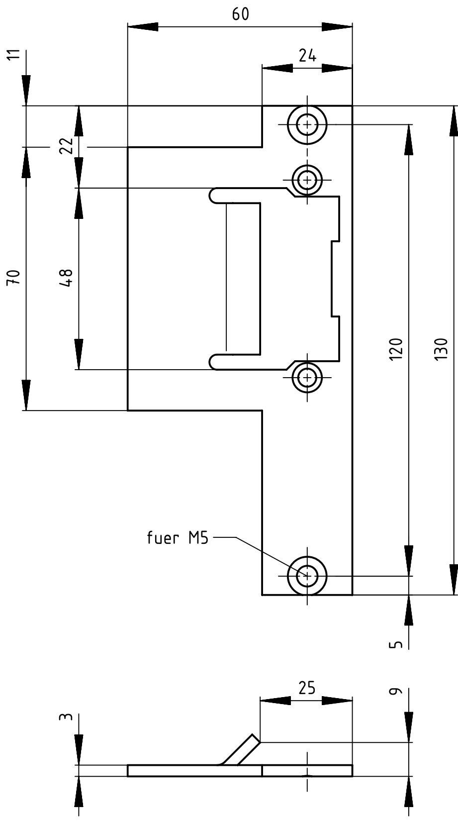
Abbildung Gehfluegel DIN links DIN rechts spiegelbildgleich
