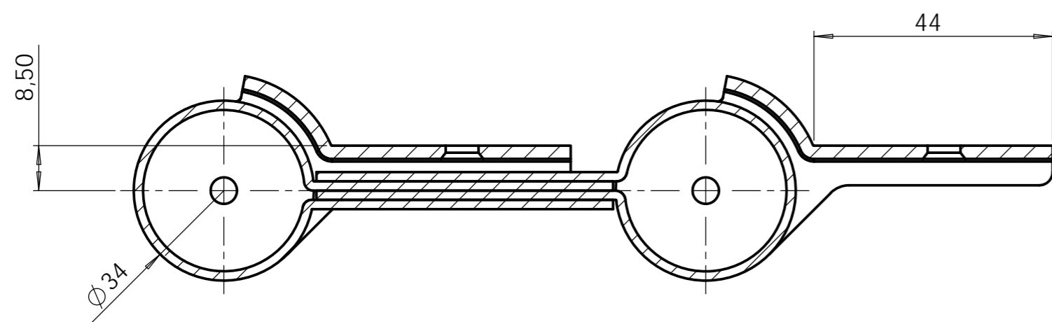
SCHNITT A-A
