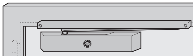
T46G: Gegenbandseitige Türblattmontage
