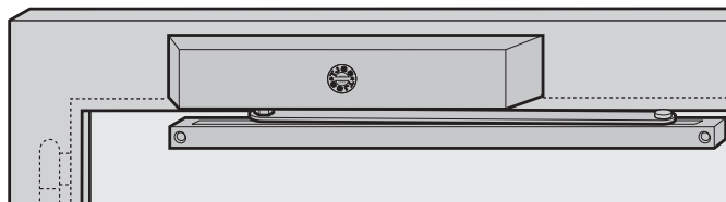
T46: Gegenbandseitige Kopfmontage
