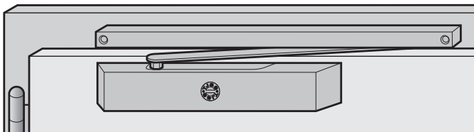
T46: Bandseitige Normalmontage
