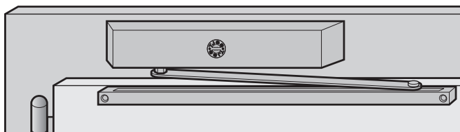
T46G: Bandseitige Kopfmontage
