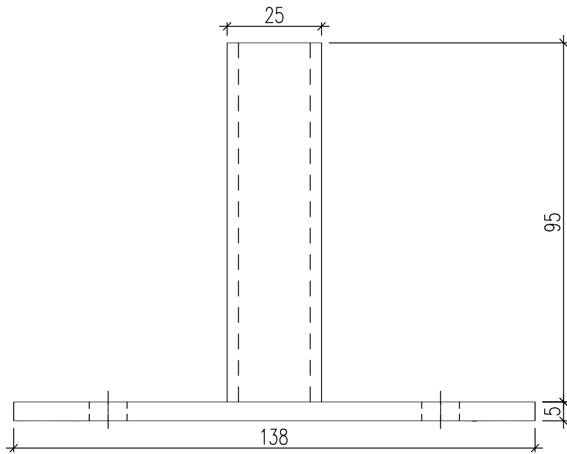
Seitenansicht
