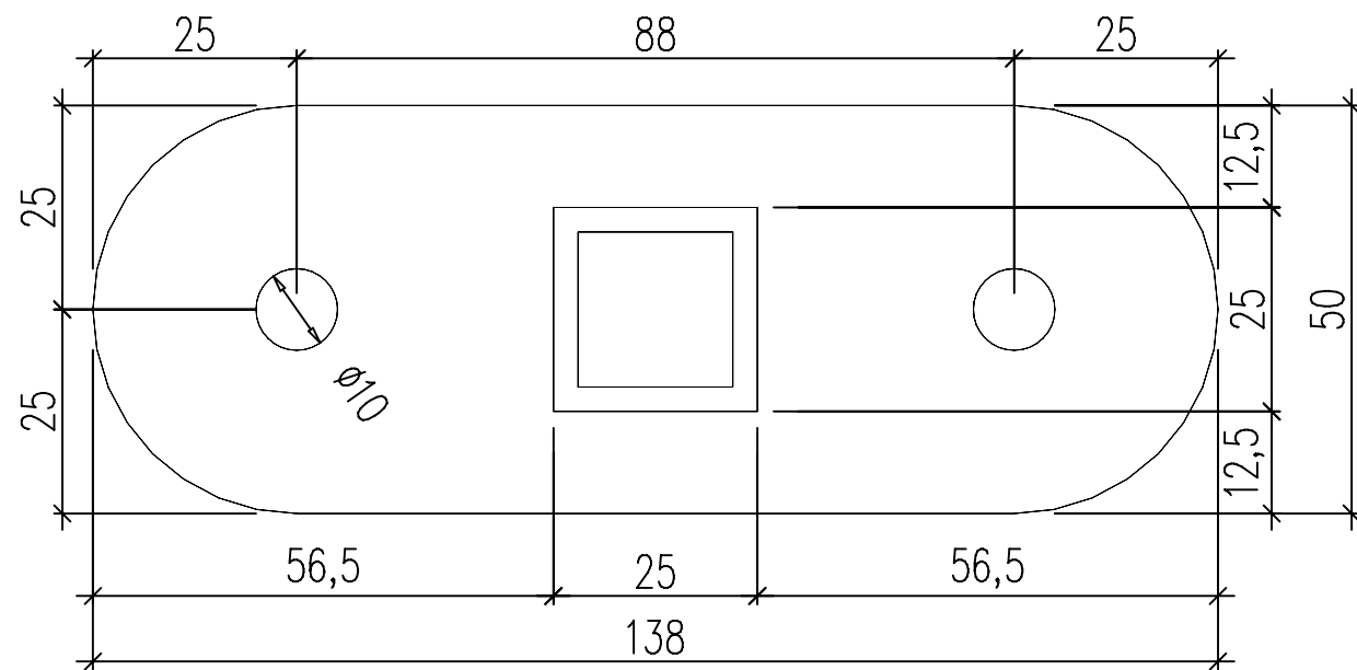
Draufsicht
