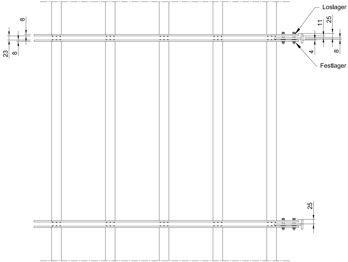
Draufsicht
