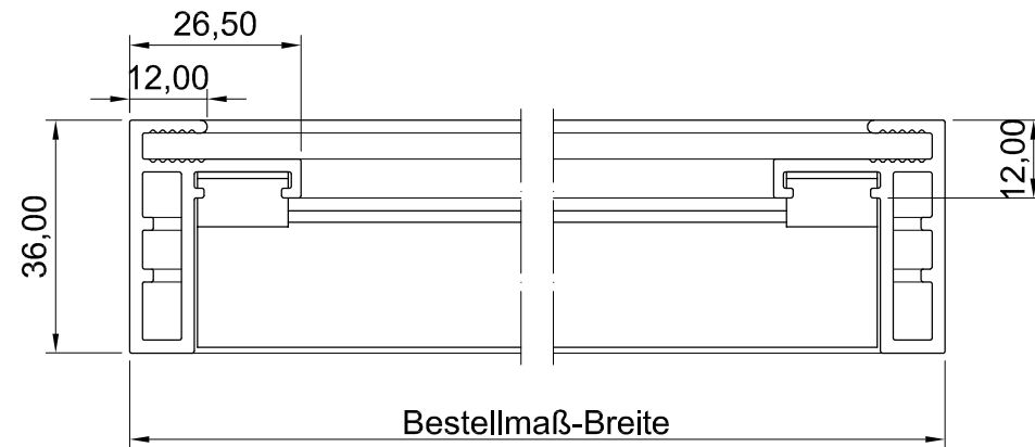
Draufsicht
