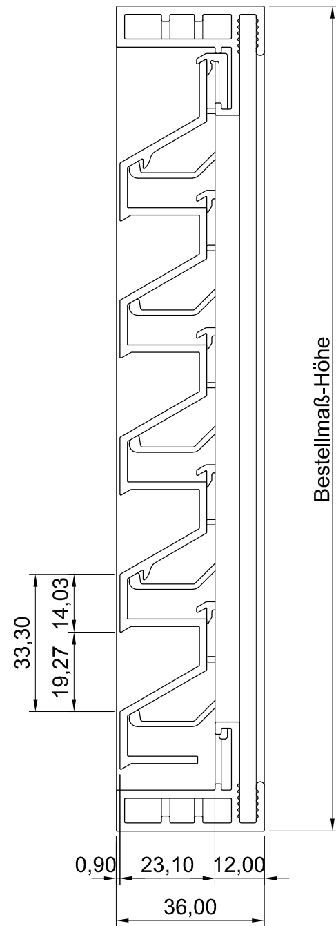
Vorderansicht
