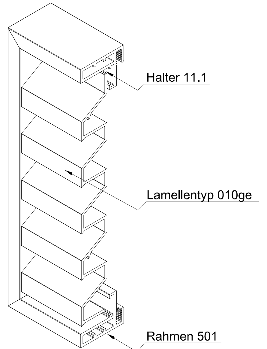
ISO-Ansicht
