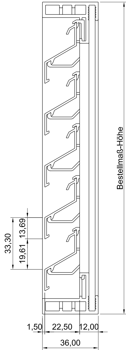
Seitenansicht
