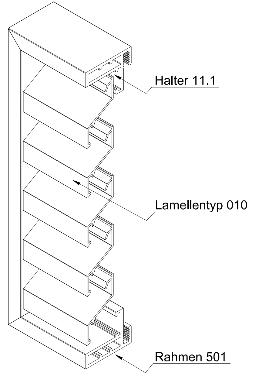
ISO-Ansicht
