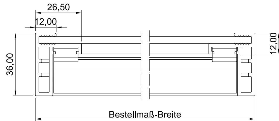
Draufsicht
