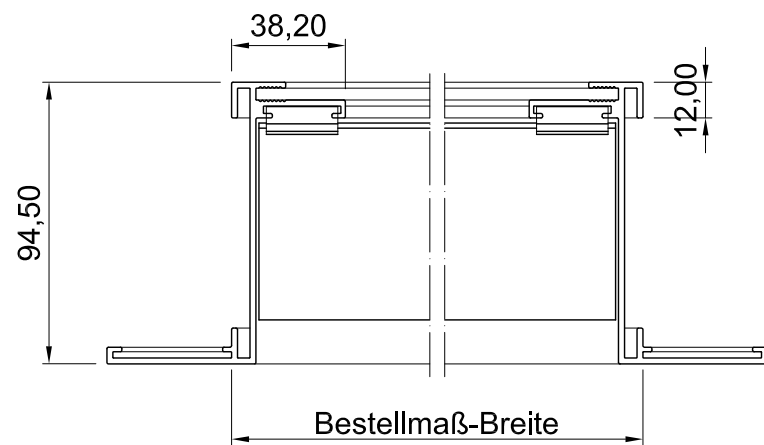
Draufsicht
