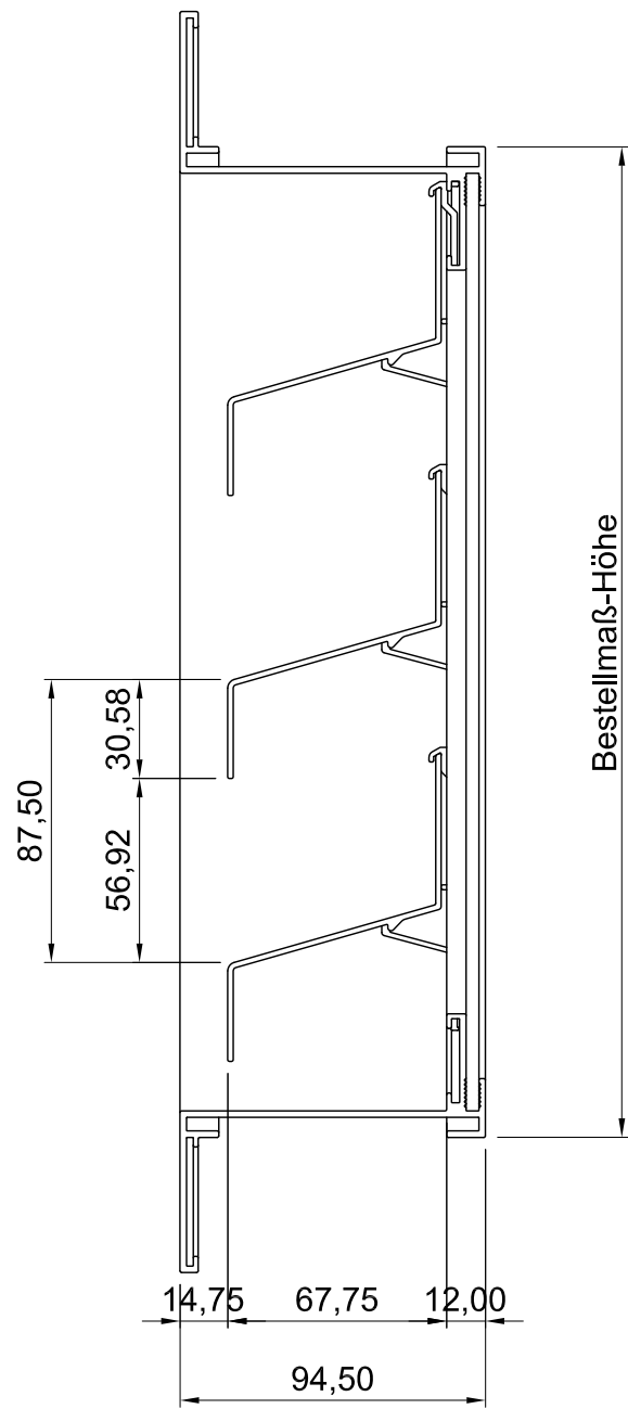
Seitenansicht
