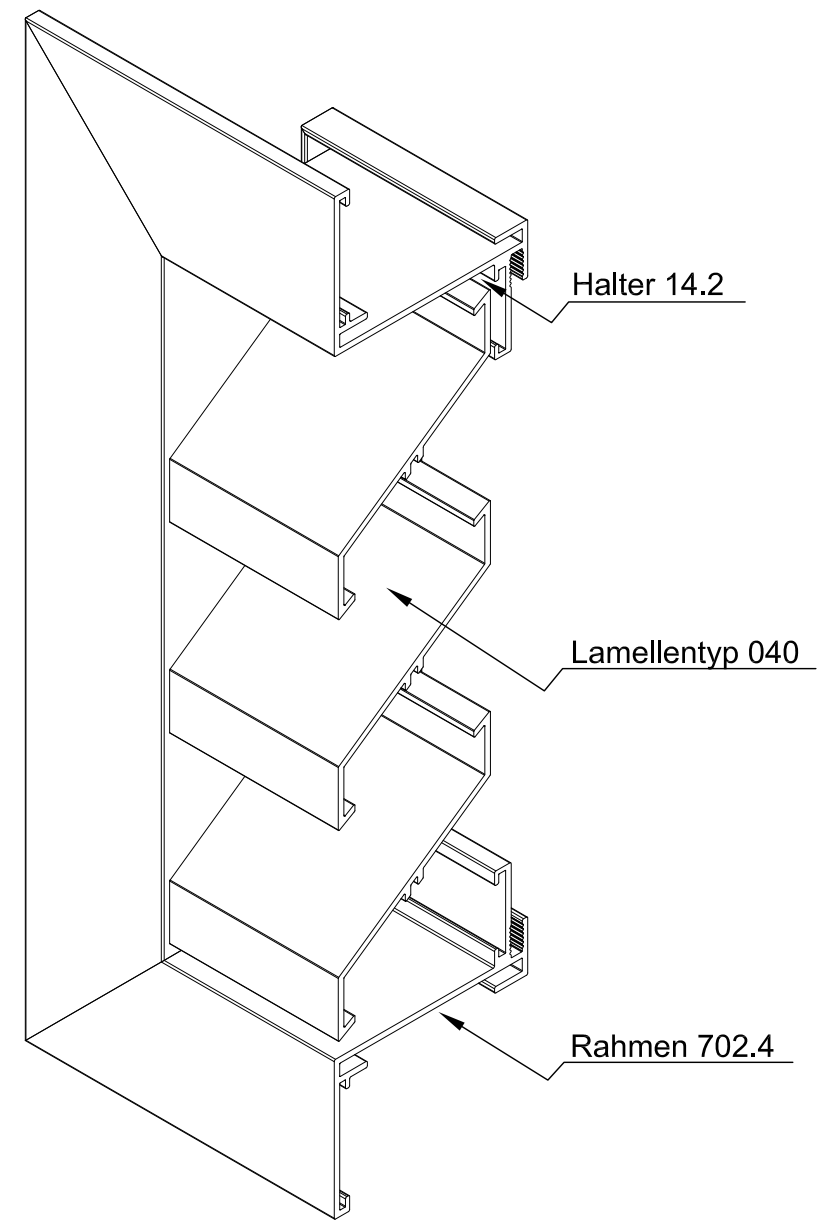
ISO-Ansicht
