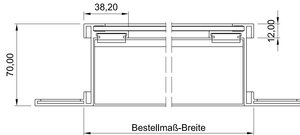
Draufsicht
