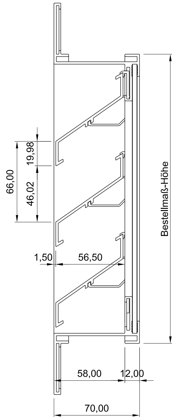
Seitenansicht
