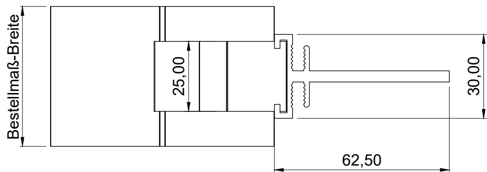
Draufsicht
