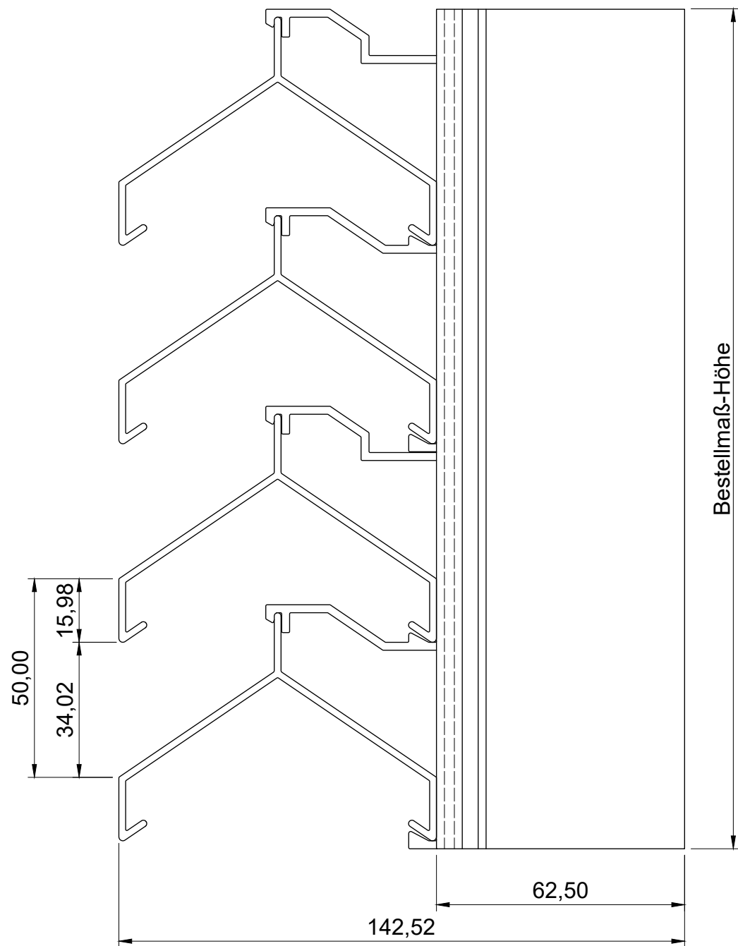
Draufsicht
