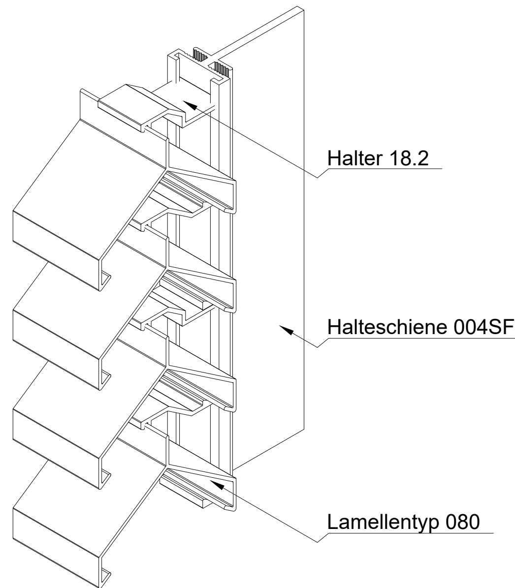
ISO-Ansicht
