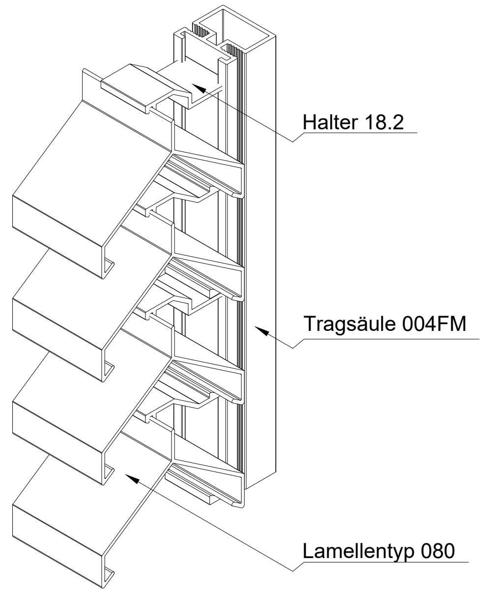
ISO-Ansicht
