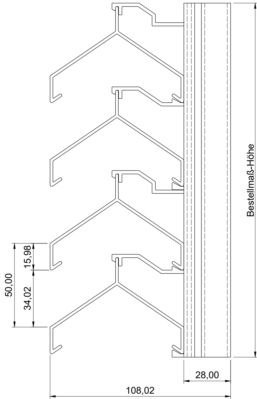
Draufsicht
