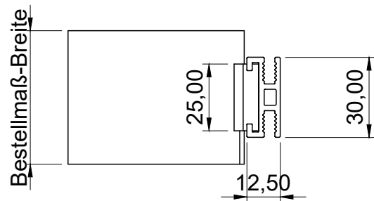
Draufsicht
