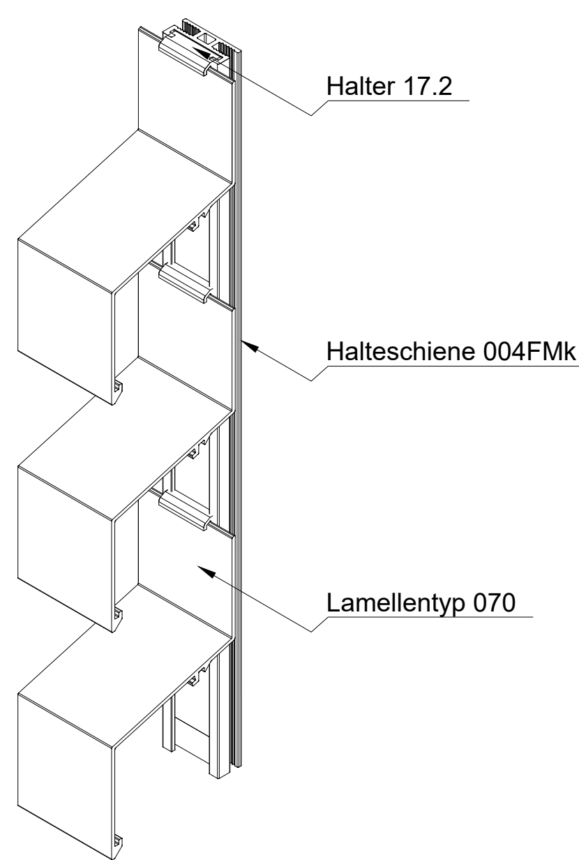
ISO-Ansicht
