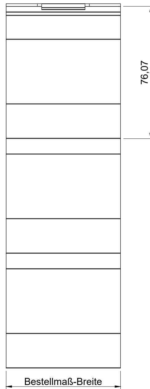
Seitenansicht
