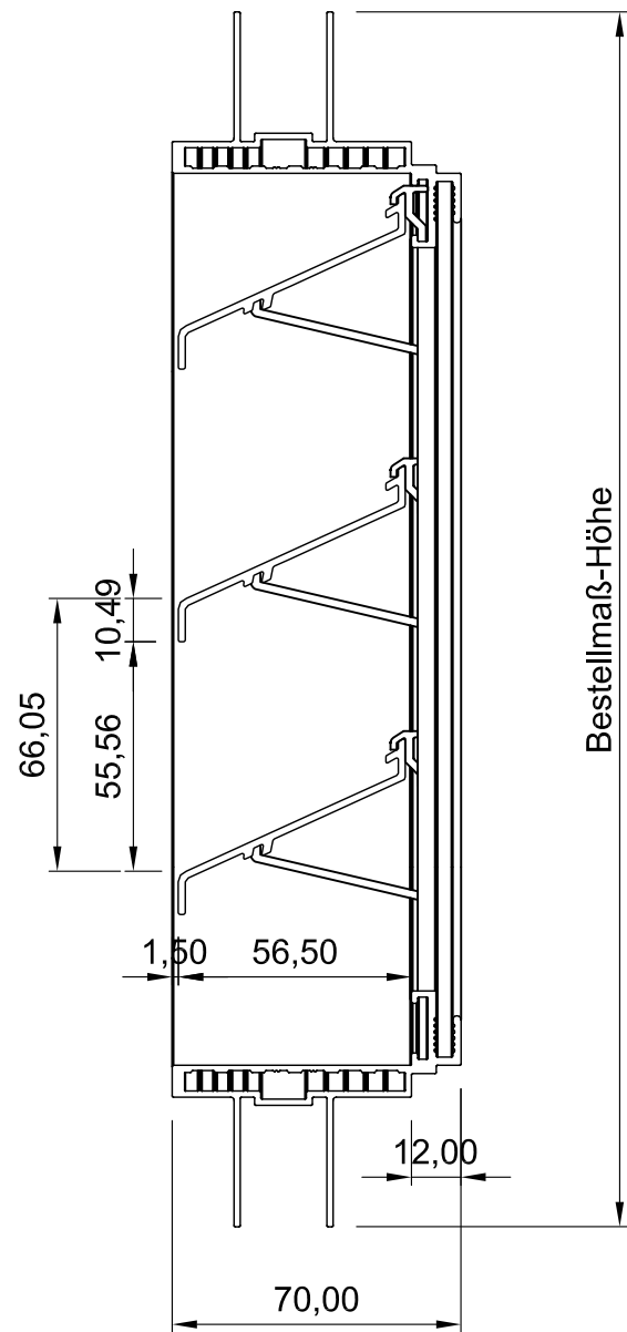
Seitenansicht
