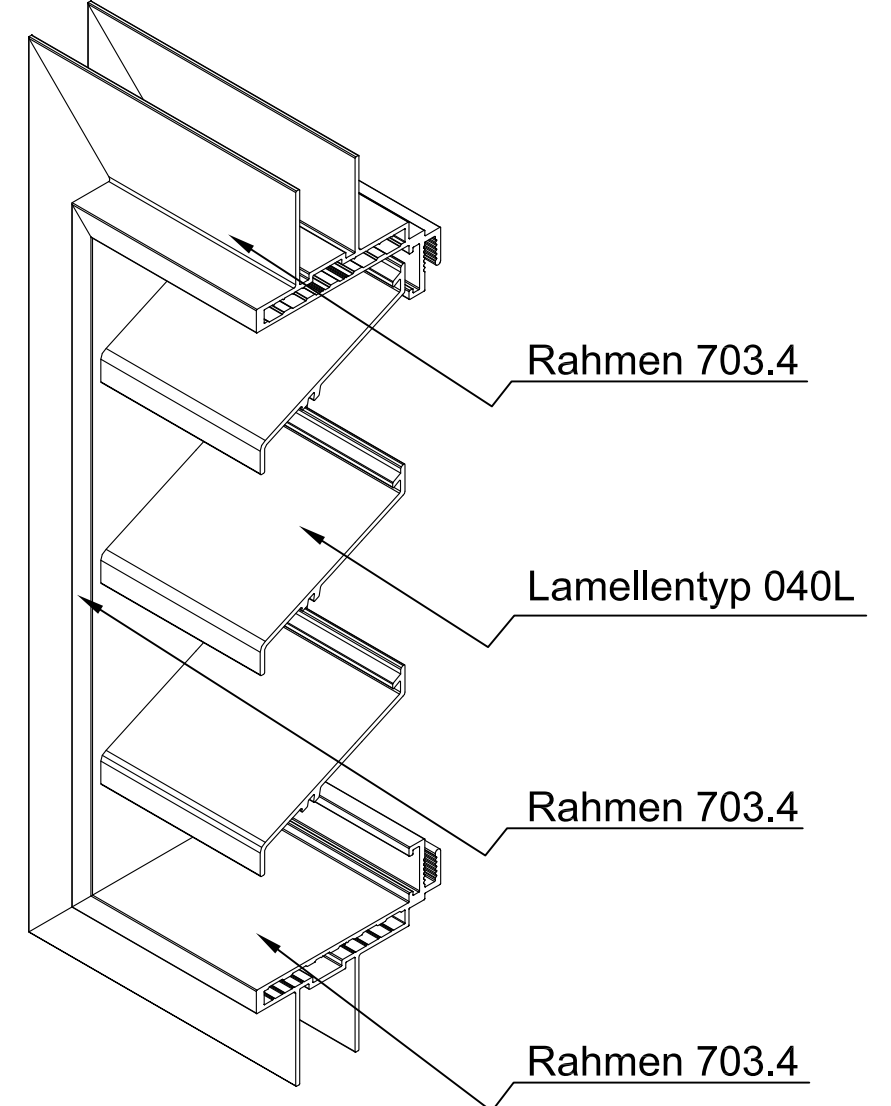
ISO-Ansicht
