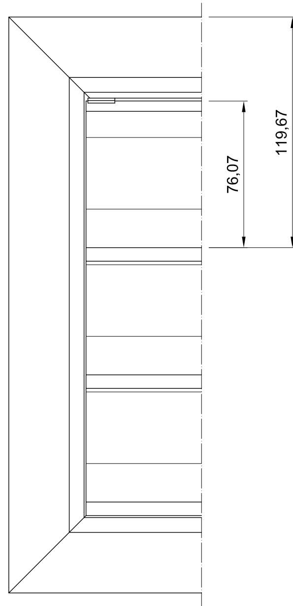
Vorderansicht
