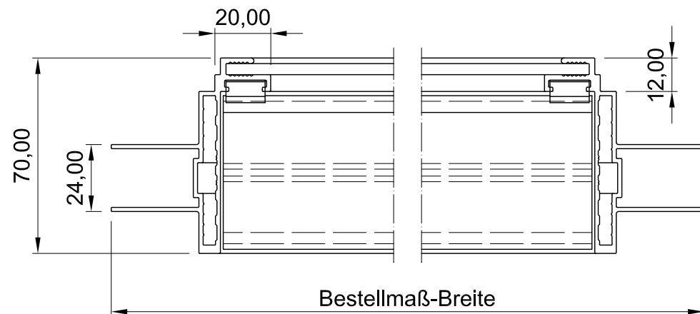
Draufsicht
