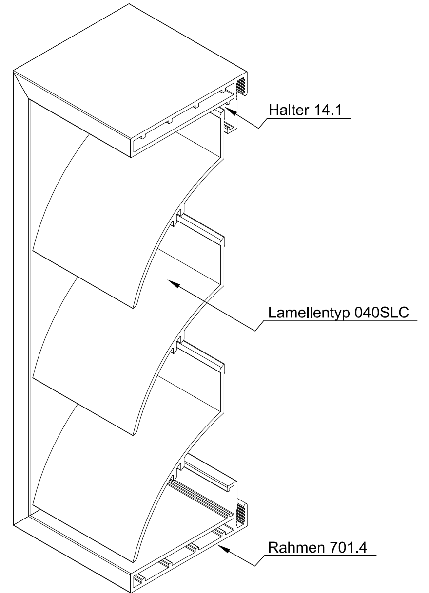
ISO-Ansicht
