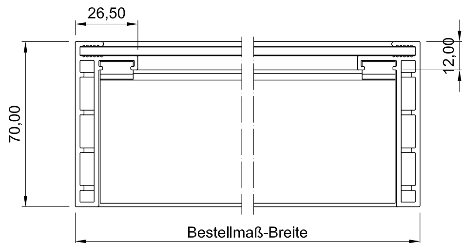
Draufsicht
