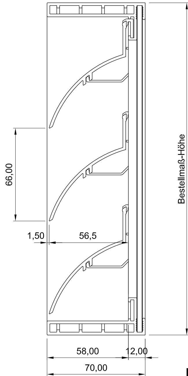
Seitenansicht
