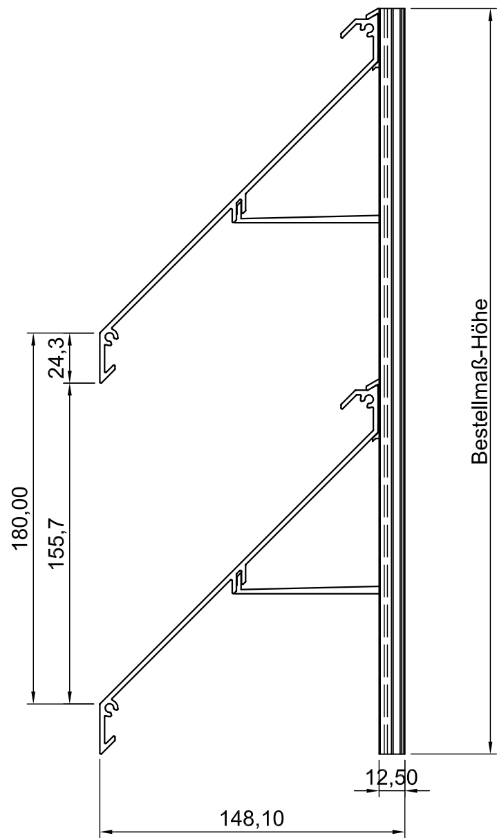
Seitenansicht
