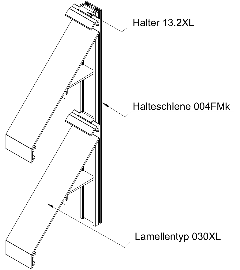
ISO-Ansicht
