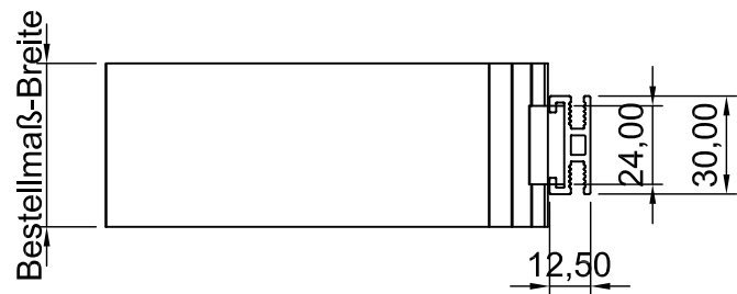
Draufsicht
