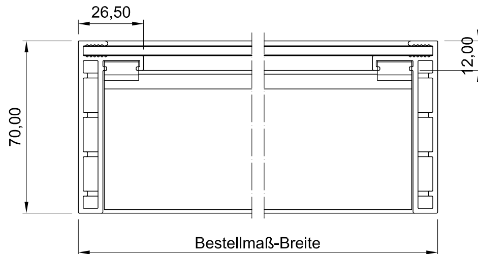
Draufsicht
