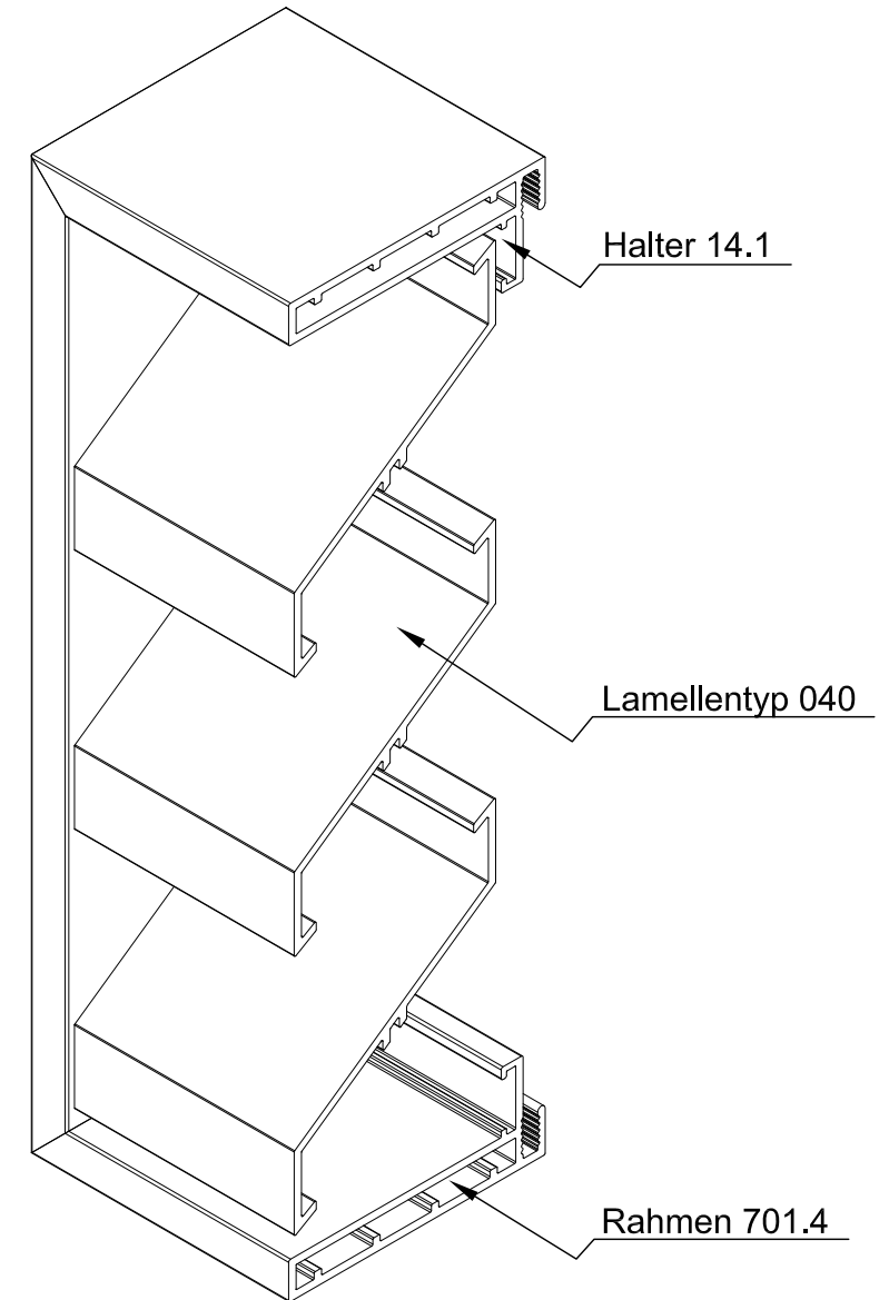
ISO-Ansicht
