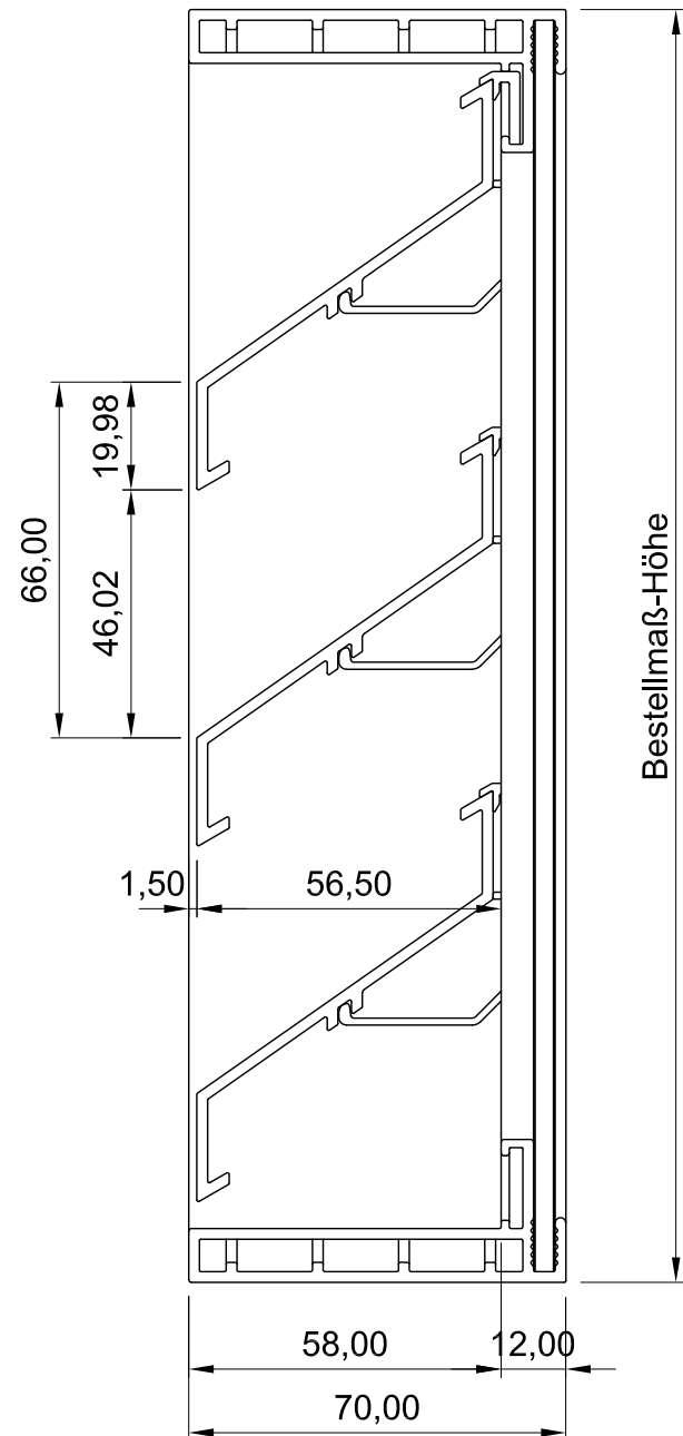
Seitenansicht
