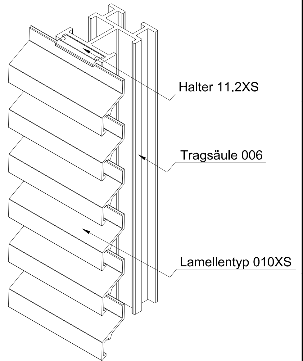
ISO-Ansicht
