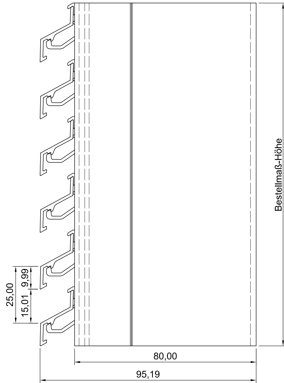
Draufsicht
