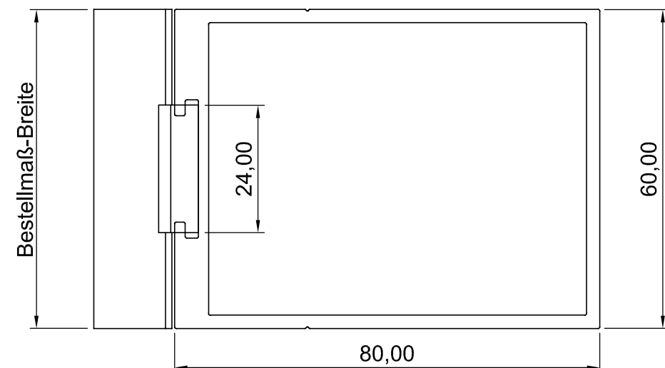
Draufsicht
