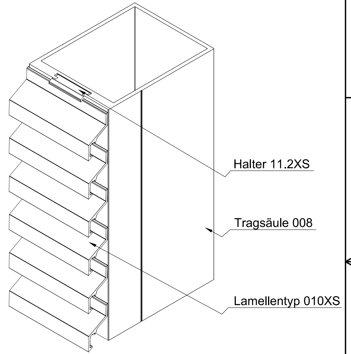
ISO-Ansicht
