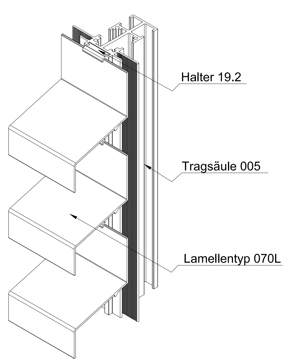
ISO-Ansicht
