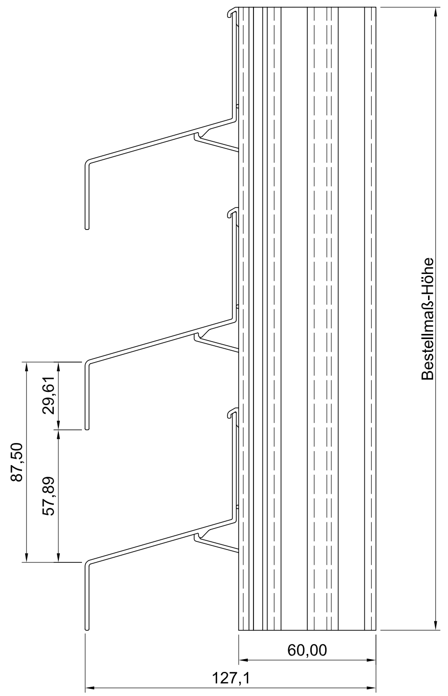
Draufsicht
