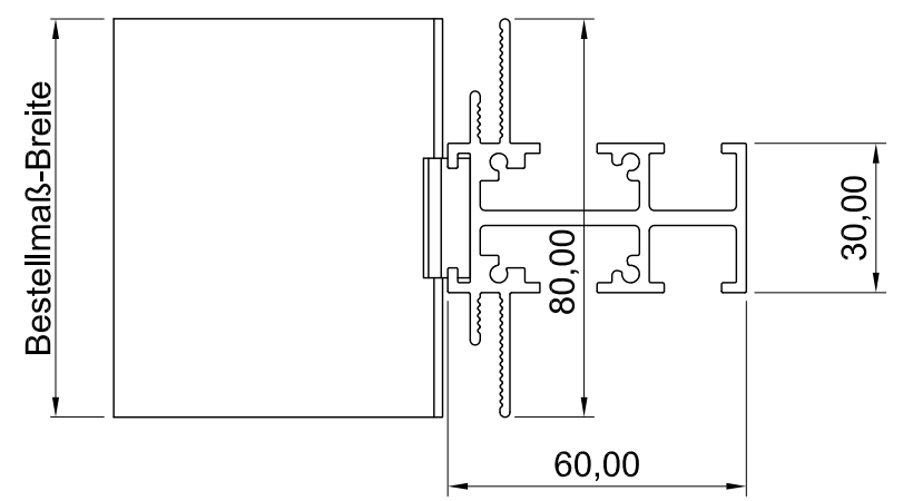
Draufsicht
