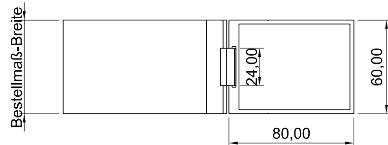
Draufsicht
