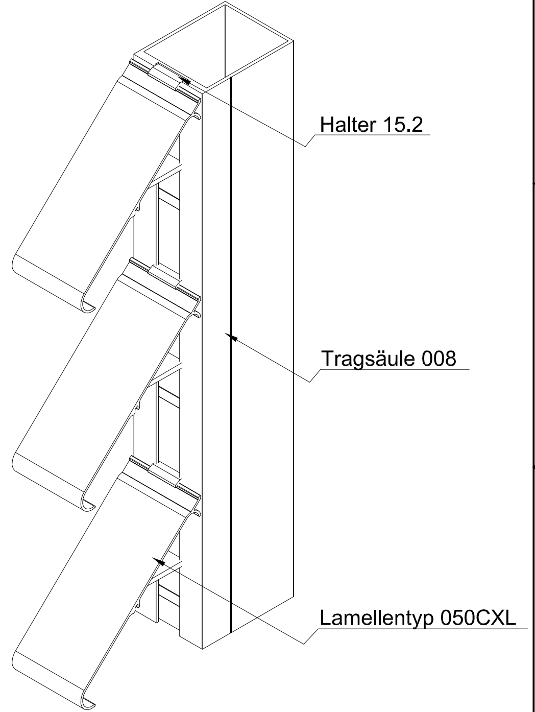
ISO-Ansicht
