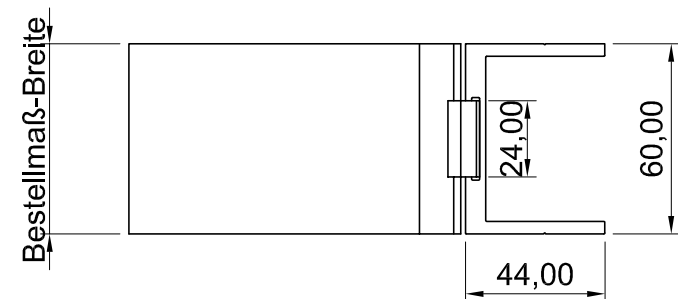
Draufsicht
