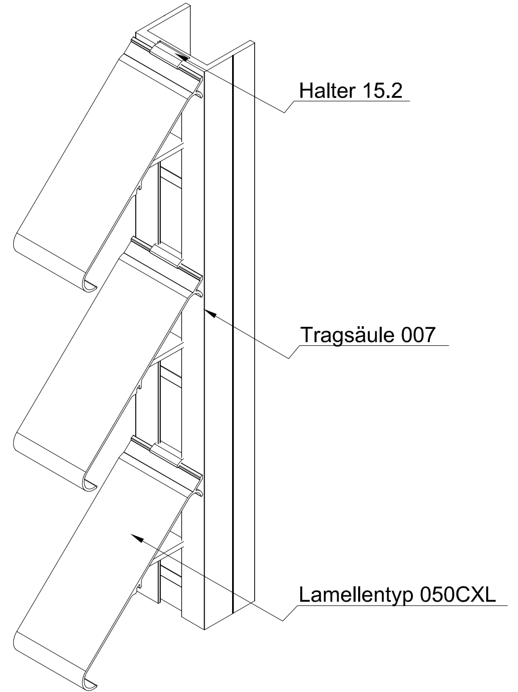
ISO-Ansicht
