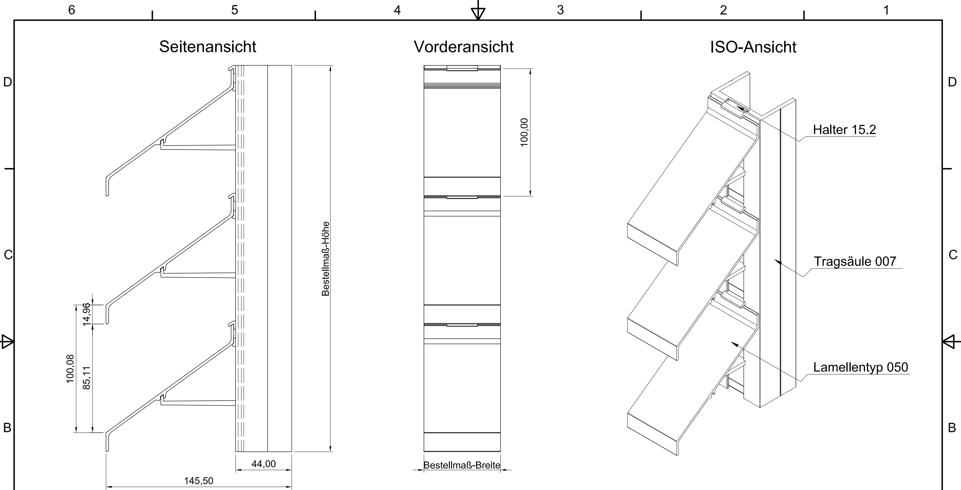
MLL-TYP 757 freier Lüftungsquerschnitt 69%
